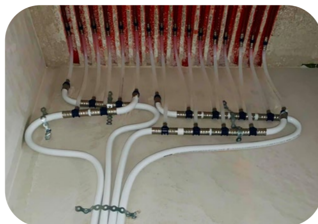
Deska po odstranění bedněni, s Tichelmannovým připojením vedeným na stěně a připojením panelů Wavin Comfia CW-90
