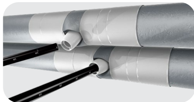
Připojení panelů chladicího stropu k rozdělovači
