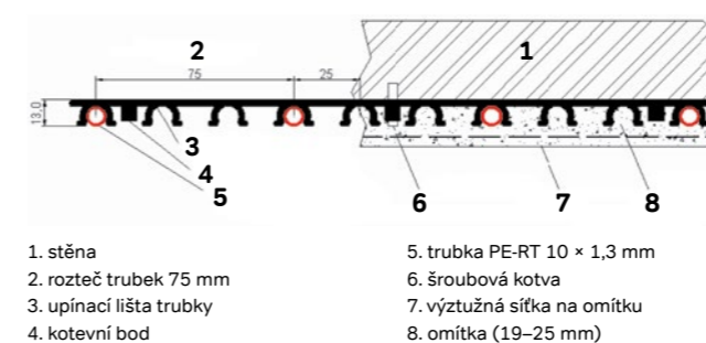
Konstrukce stěny s Wavin Comfia WW-10
