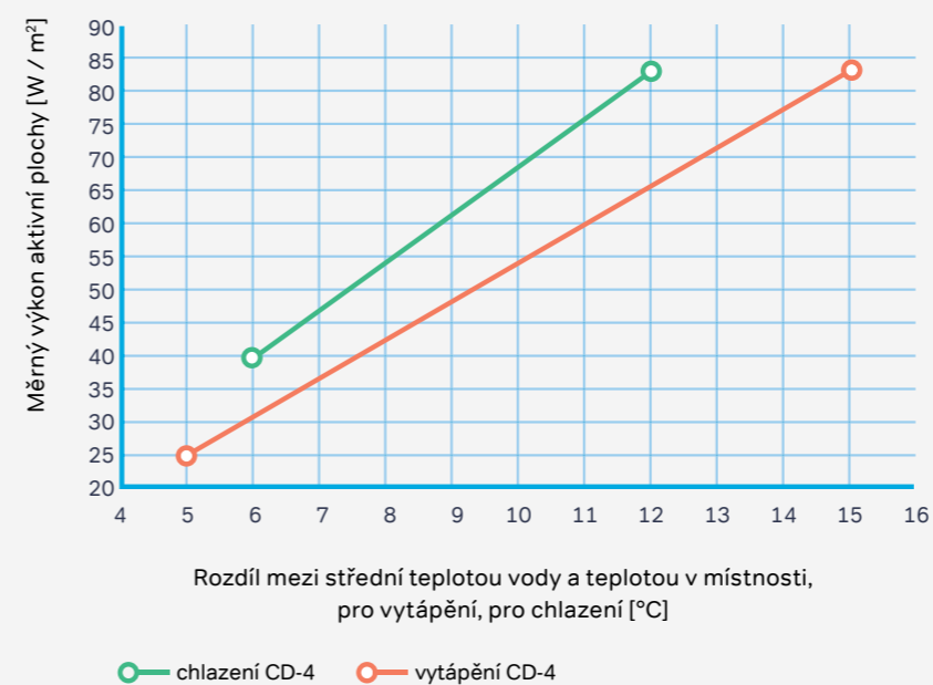
Výkonový diagram systém vytápění a chlazení Wavin Comfia CD-4
