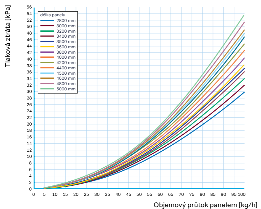
Diagram tlakových ztrát panelů Wavin Comfia CD-4
