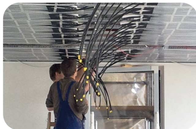
Připojení panelů chladicího stropu k rozdělovači
