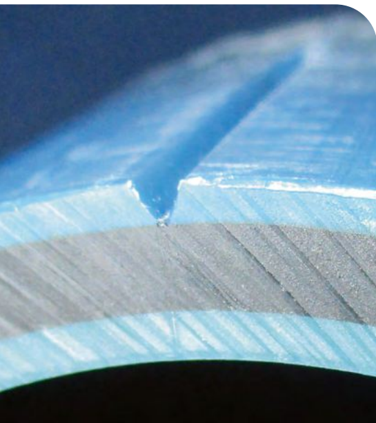
Abbildungen aus EN ISO 13479 und Wavin TS DOQ ® Prüfstück bei Hessel Ingenieurtechnik, Roetgen (NPT+-Test, 2017)
