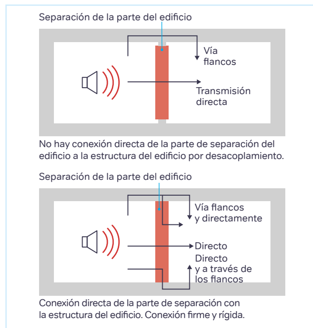
Figura 7: Información sobre las posibles rutas de transmisión para diferentes elementos de la construcción.
