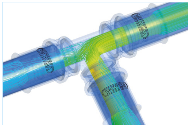
Figura 10: Condiciones de flujo en una T.
