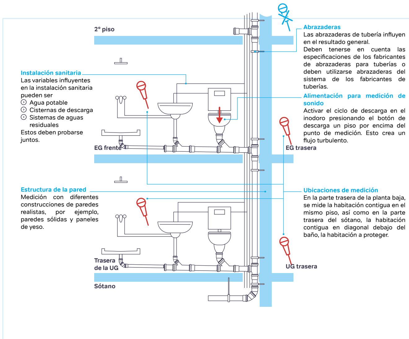
Figura 47: Configuración representativa para una medición en condiciones reales.
