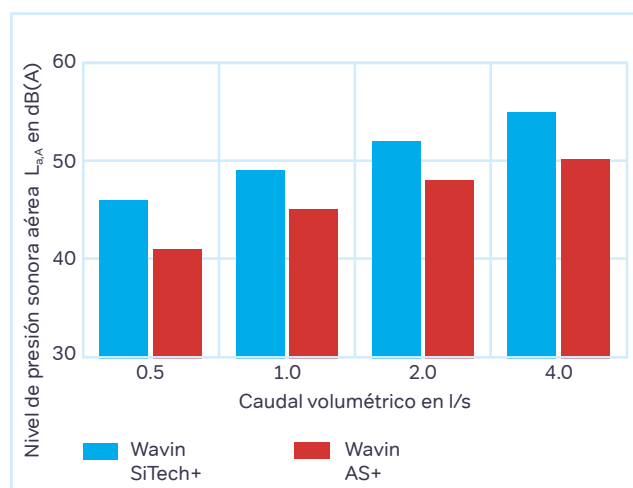
Figura 46: Influencia de la calidad de la tubería en la presión sonora aérea nivel.
