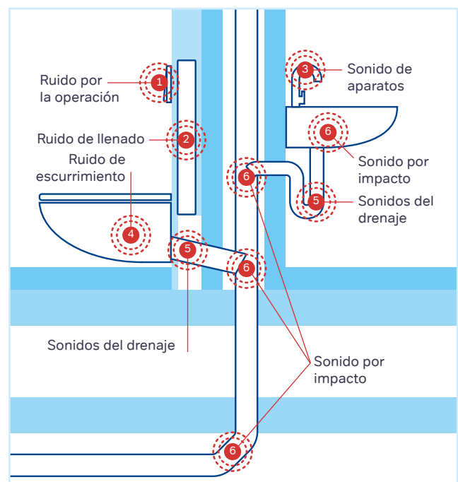
Figura 18: Fuentes de ruido en instalaciones de agua potable y sanitaria.
