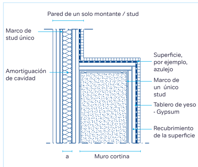
Figura 29: Muro de entramado simple con instalación de muro cortina adicional.
