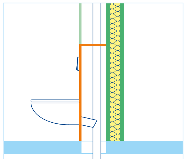
Figura 32: Instalación de muro cortina frente un panel de yeso (basado en fuente 8)
