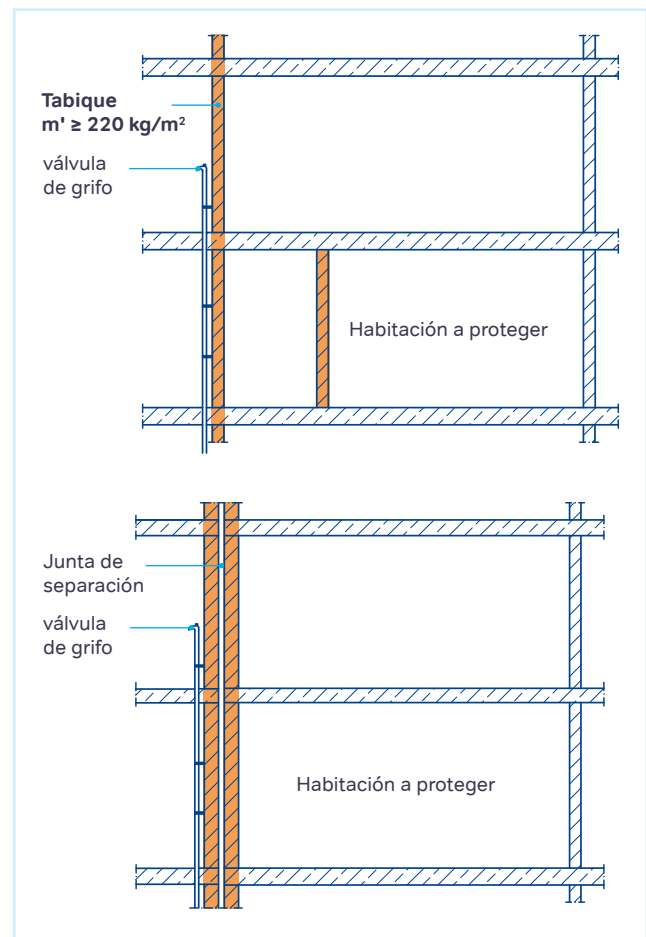
Figura 28: Disposición de los accesorios del grupo de accesorios II.
