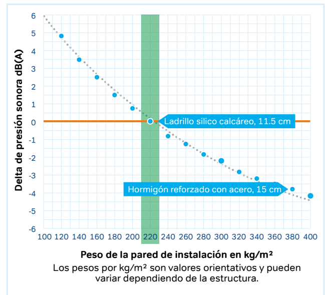
Figura 23: Ilustración del cambio en el nivel de presión de sonido en el adyacente cuarto de centavo como una función de diferentes materiales de pared de Wavin SoundCheck.
