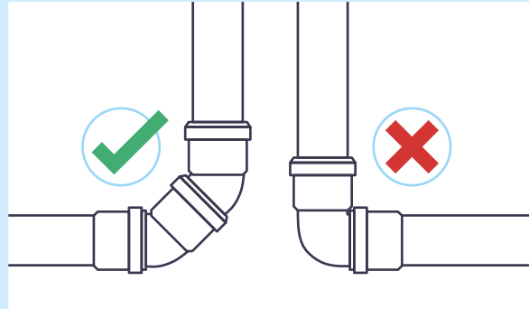
Figura 25: Situación de instalación con diferentes codos.
