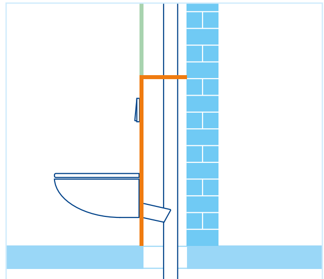
Figura 31: Muro cortina de paneles de yeso frente a muro sólido (basado en la fuente 8)
