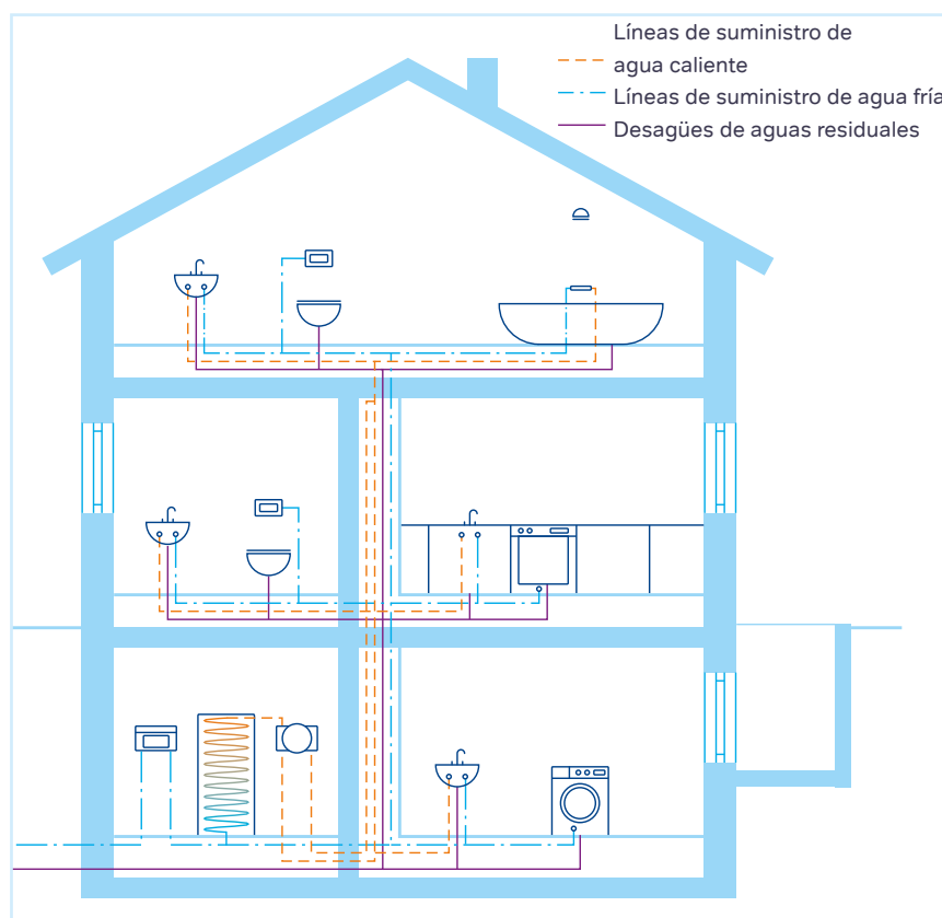
Figura 15: Líneas de suministro y eliminación en un edificio.
