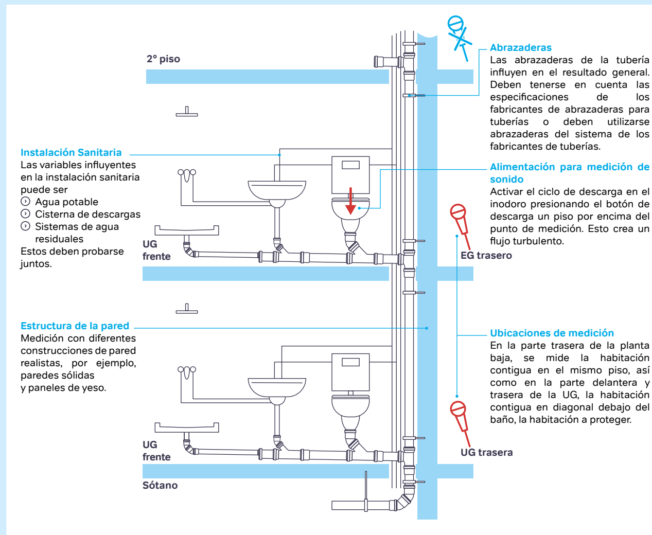
Figura 9: Configuración representativa para una medición en condiciones reales.
