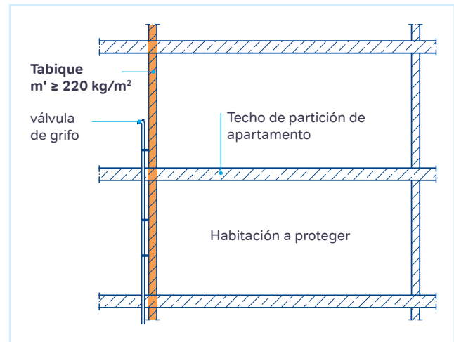
Figura 27: Disposición de los accesorios del grupo de accesorios I
