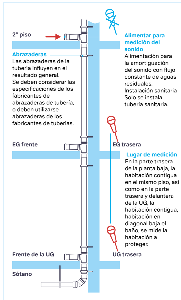
Figura 45: Configuración de medición según DIN EN 14366.
