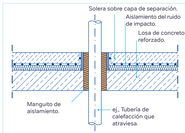
Figura 19: Pasamuros sin puente de sonido.
