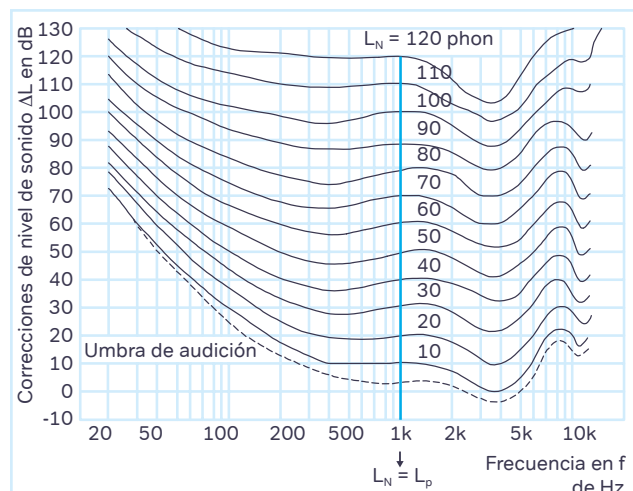
Figura 4: Conexión entre volumen de sonido percibido subjetivamente L_N y nivel de presión acústica medible objetivamente L_p . L_N y L_p solo coinciden en la frecuencia f=1000 Hz.
