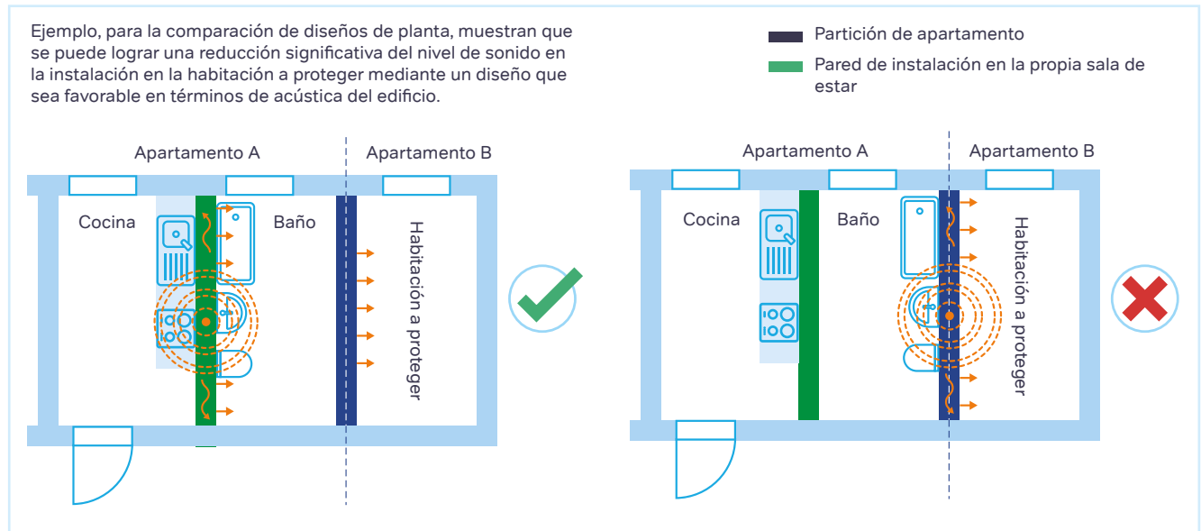
Figura 22: Una planta favorable desde el punto de vista de acústica del edificio.
