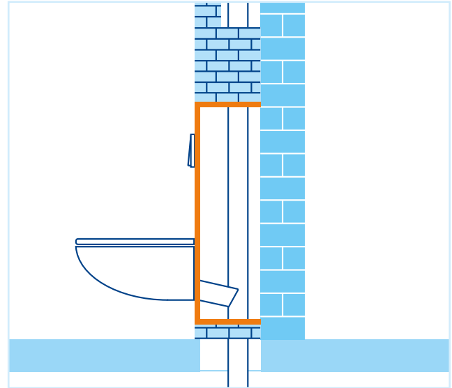
Figura 30: Muro en construcción húmeda frente a muro macizo (basado en la fuente 8)
