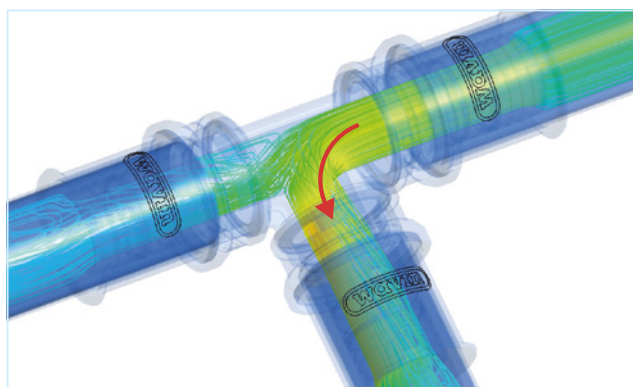
Figura 34: Condiciones de flujo en una T.
