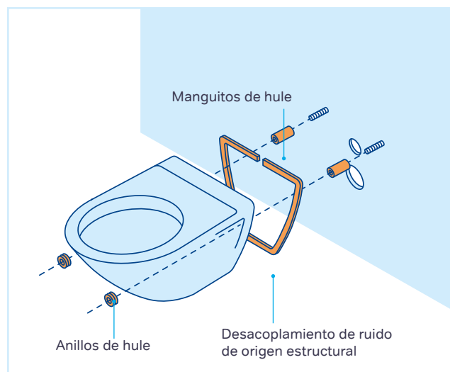
Figura 26: Diseño de un sistema de inodoro suspendido sin puentes de sonido.
