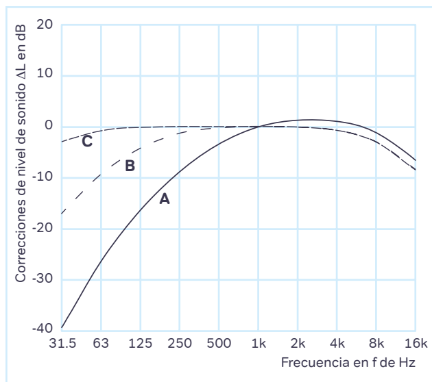
Figura 2: Corrección del nivel de presión sonora L según DIN EN ISO 16032 (o DIN EN 60651 retirado) para clasificaciones A, B y C.
