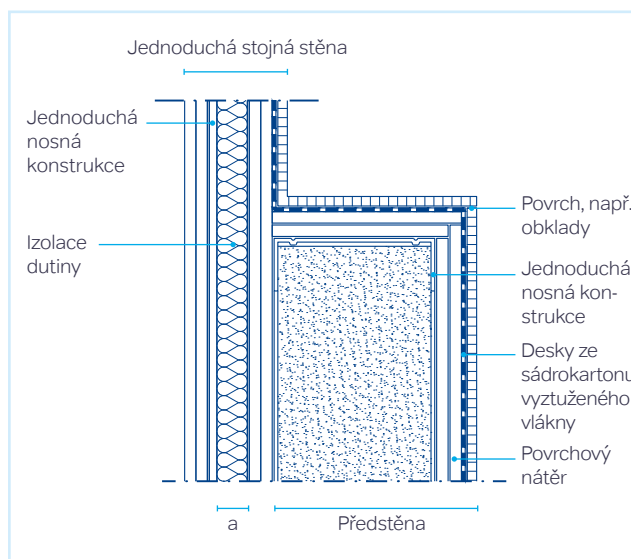
Obrázek 29: Jednoduchá stojná stěna s přídatnou instalací v předstěně
