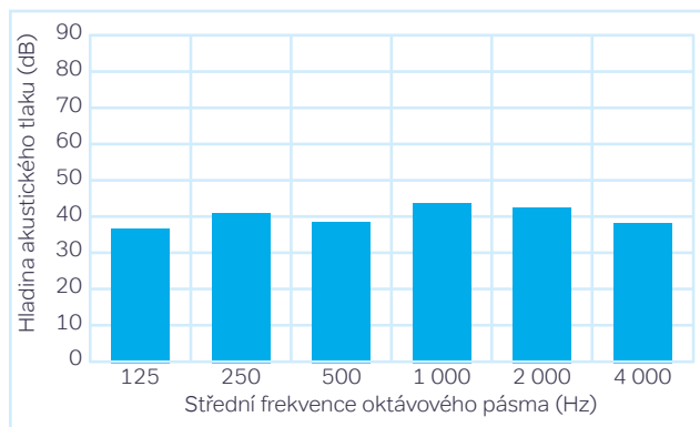
Obrázek 5: Oktávové spektrum
