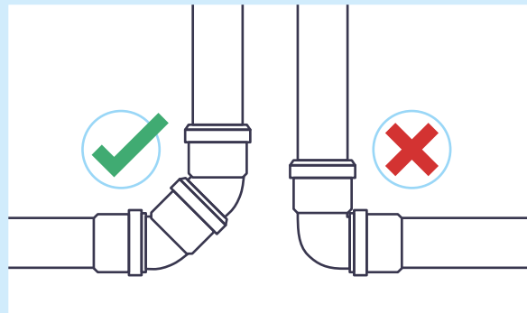
Obrázek 25: Montážní rozdíl mezi různými tvary kolen
