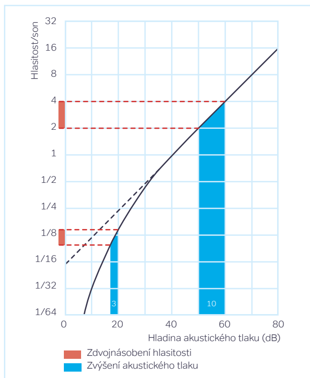
Obrázek 6: Subjektivní vnímání hlasitosti podle Zwicklera
