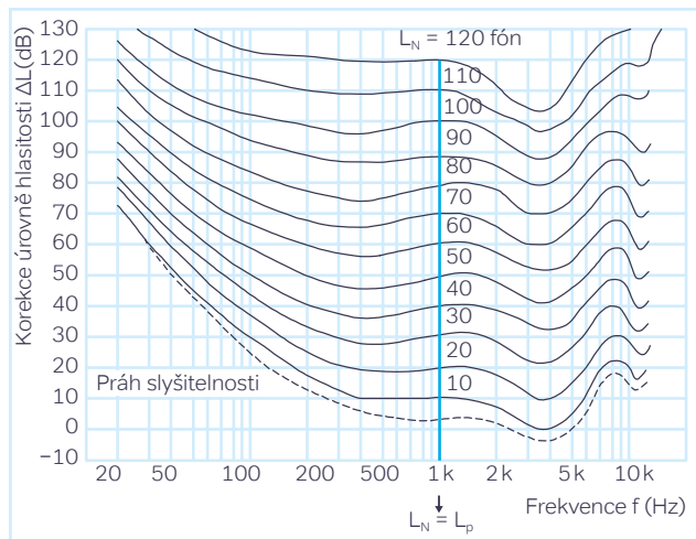
Obrázek 4: Souvislost mezi subjektivně vnímanou úrovní hlasitosti L_N a objektivně měřitelnou hladinou akustického tlaku L_p . Shoda mezi L_N a L_p platí pouze při frekvenci f = 1\ 000\ \text{Hz} .
