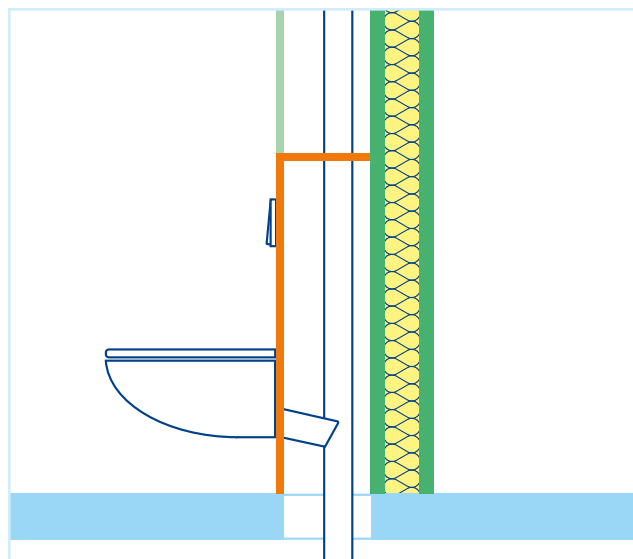
Obrázek 32: Instalace předstěny před suchou stěnou (s odkazem na zdroj č. 8)
