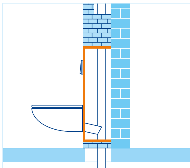
Obrázek 30: Obezdní mokrou konstrukcí před robustní stěnou (s odkazem na zdroj 8)
