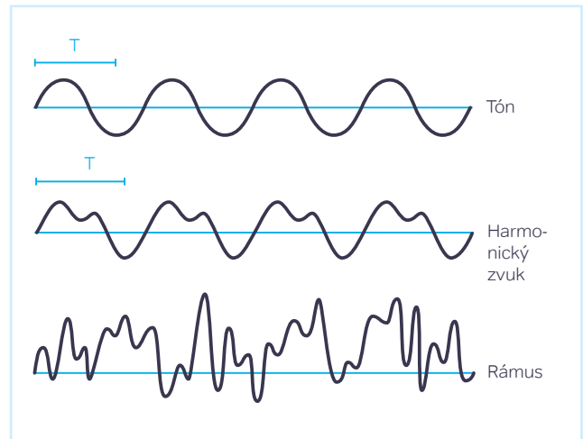
Obrázek 13: Tón – harmonický zvuk – rámus
