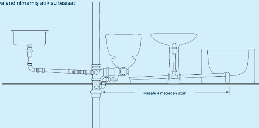
Şekil 4: Uygulama örneği: Ana kolon ile atık su noktası arası 4 metreden uzun ise branşman hattında da otomatik havalık şapkası kullanılmalıdır (a).
