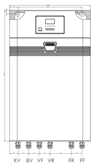
Tilslutningsskitse, højrevendt
