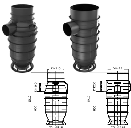
Uliční vpust Tegra se sifonem a filtrem
