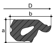
Těsnění – pro Tegrú 1000 1. generace
