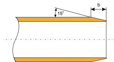
Rozměry úkosu
