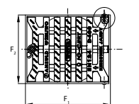
Litinná mříž D400 Ø 315 mm – do teleskopické roury
