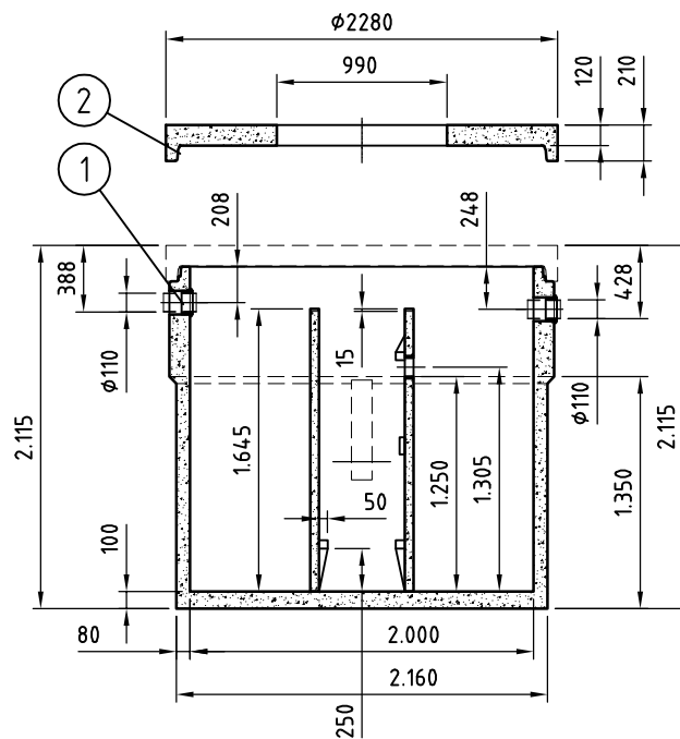
Snede A-A'
