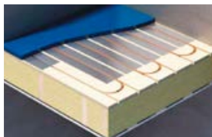
Exempelbild på installation på spårad aluminium plåtar.
