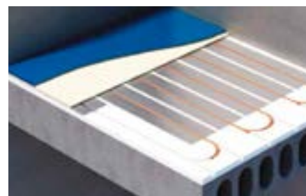
Exempelbild på installation på EPS skiva med plåtar.
