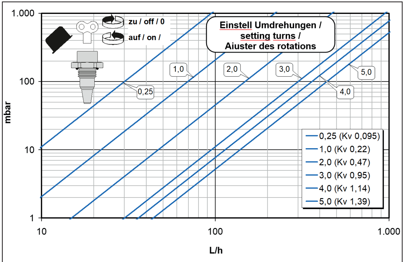
Fig(3): Diagram som visar den uppnåbara flödes hastigheten baserat på antalet gjorda ventilvarv
