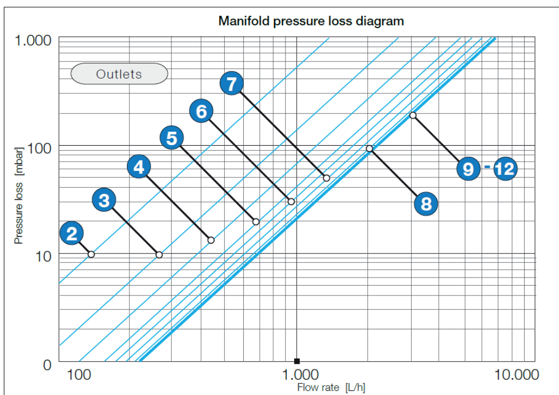
Fig(2): Diagram som visar systemets tryckförlust baserat på flödet, för alla fördelarstorlekar
