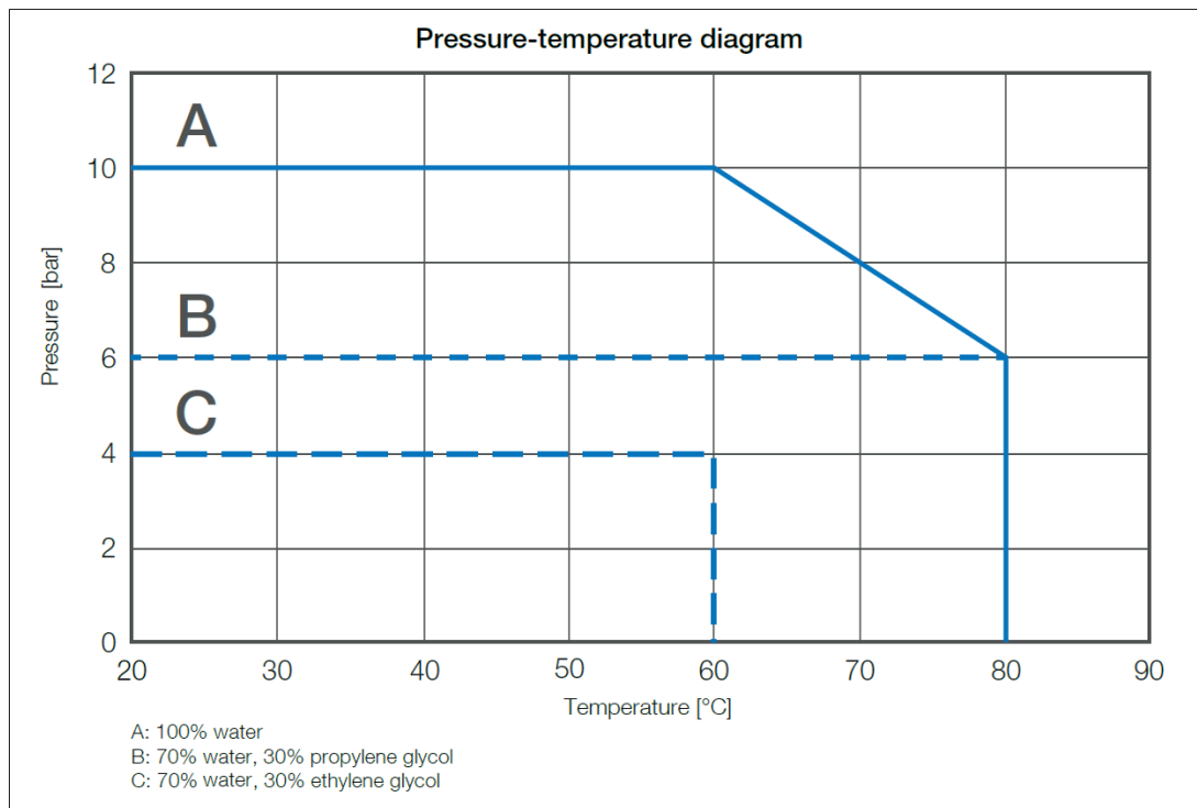
Fig(1): Diagram som visar det maximalt tillåtna systemtrycket baserat på systemets temperaturer
