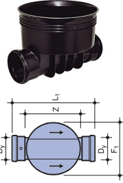
Basic 400 - Düz Taban
