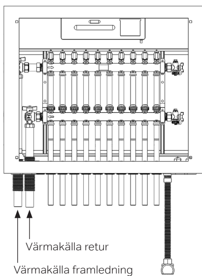
Anslutningsskiss Vänster
