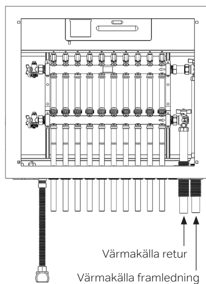
Anslutningsskiss Höger
