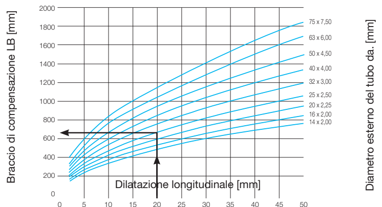
Fig.34: Calcolo del braccio di compensazione dei tubi multistrato Wavin.
