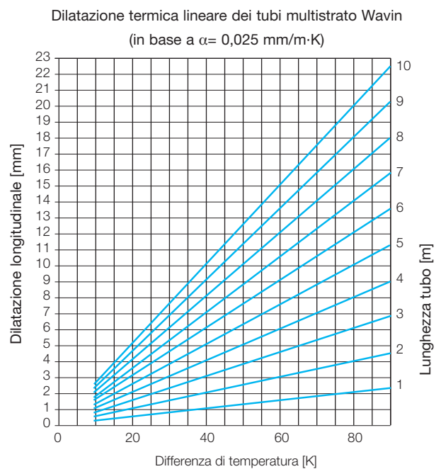
Fig. 32: Dilatazioni longitudinali dei tubi multistrato Wavin.
