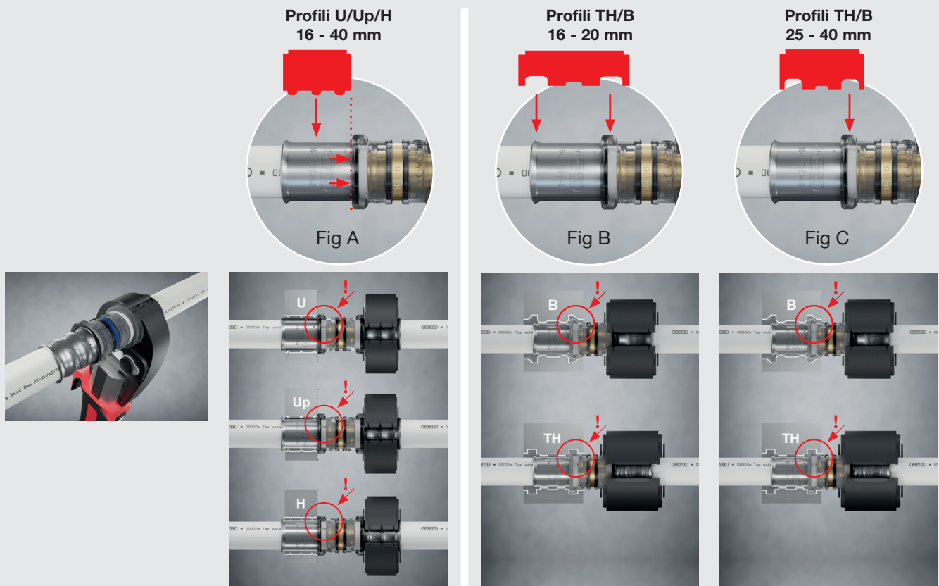
Fig. 24: Posizionamento ganasche con Tigris K5 e Tigris M5
