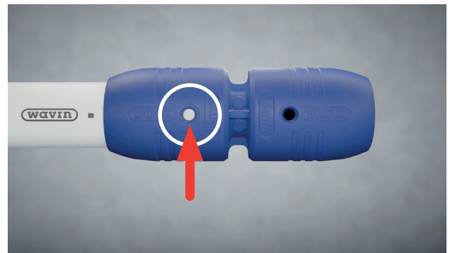
Fig.19: Attraverso la finestra di controllo della calotta si può controllare il corretto inserimento del tubo fino alla battuta
