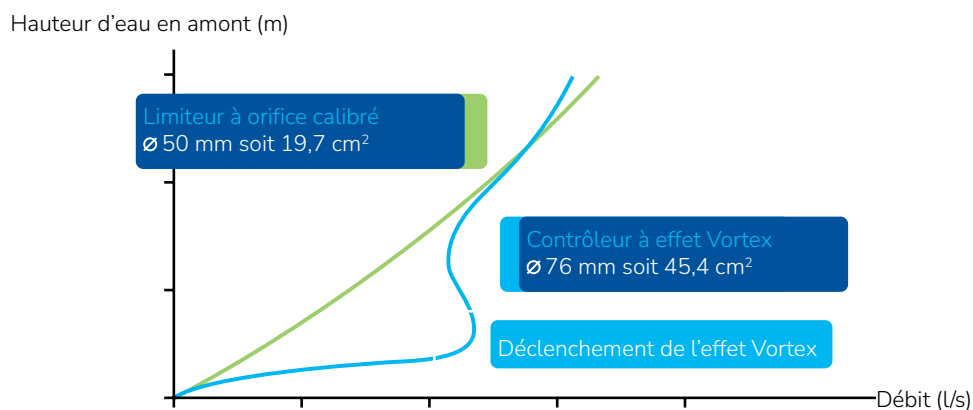
Comportement hydraulique d'un limiteur et d'un contrôleur de débit :
