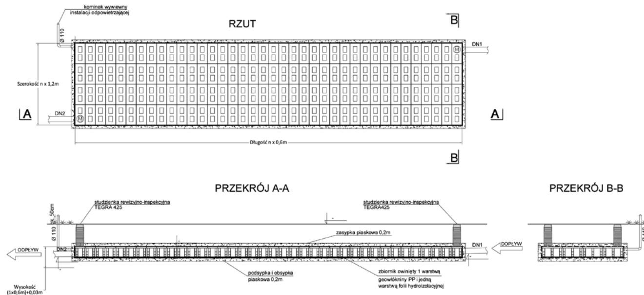
Rys. 11.1.5. Przykład zbiornika retencyjnego Wavin Q-Bic Plus oraz Wavin Q-Bic Plus LC w zabudowie jednowarstwowej.
