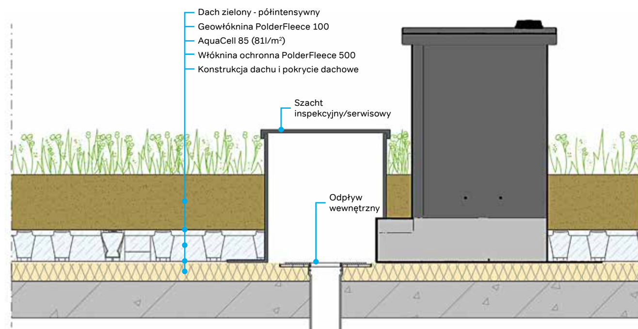
Rys. 6.1.2. Schemat dachu PolderRoof z odpływem środkowym.
