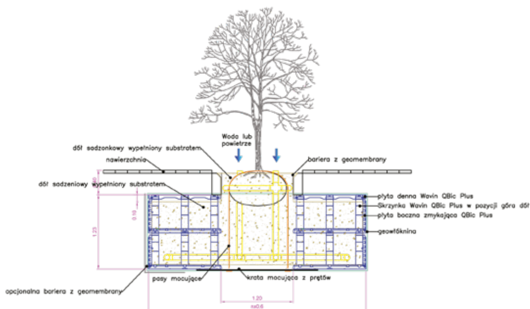
Rys. 7.5.1. Przykład montażu w zbiorniku TreeTank wysokości 1,2 m.
