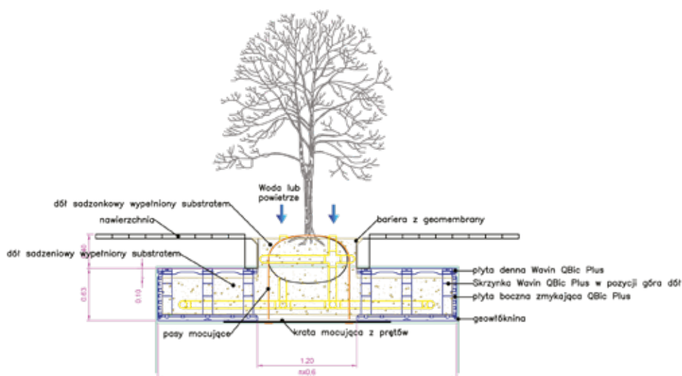
Rys. 7.5.2. Przykład montażu w zbiorniku TreeTank wysokości 0,6 m.
