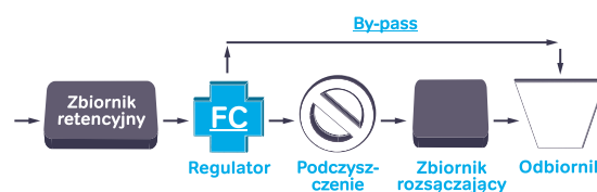
Rys. 10.1.5. Obejście by-passowe systemu podczyszczania.
