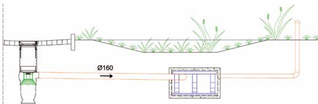
Rys 5.2. Zbiornik retencyjno-rozsączający bez możliwości inspekcji i czyszczenia współpracujący z Tegra RG, umieszczony pod niecką z nasadzoną roślinnością.
