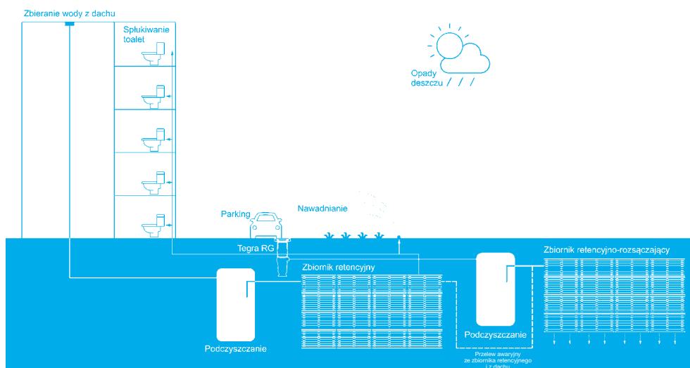
Rys 5.7. Zbieranie wody z powierzchni utwardzonych z wykorzystaniem ponownym wody deszczowej. Dodatkowo przelew awaryjny do zbiornika retencyjno-rozsączającego
