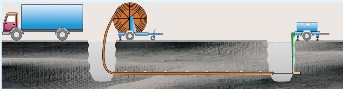
Zábor místa během instalace potrubí Compact Pipe
