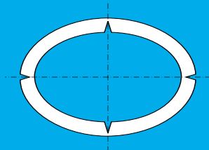
Stav starého potrubí III Labilní konstrukce potrubí-půda
