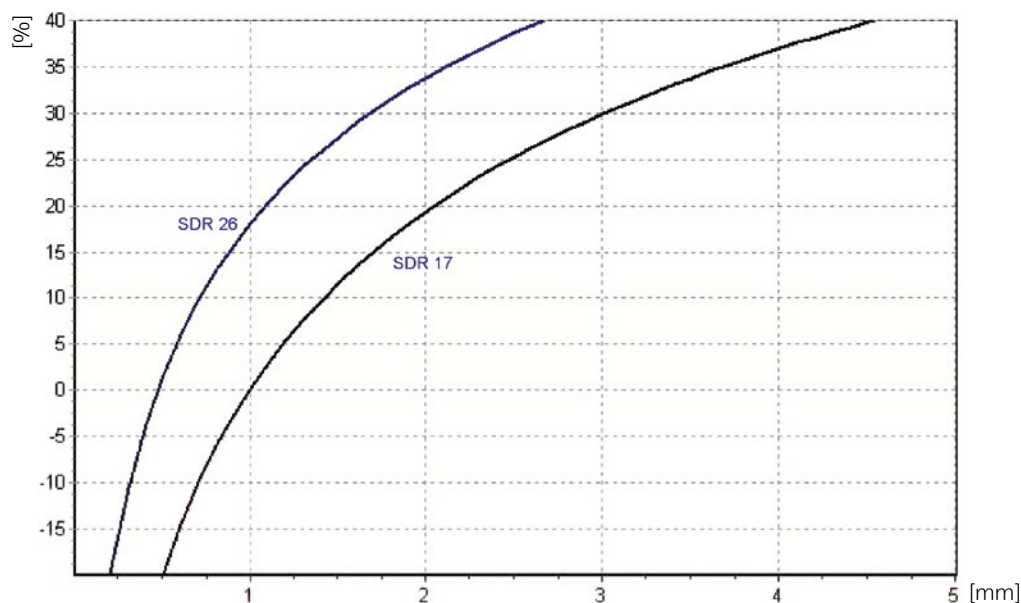
Závislost změny kapacity potrubí po sanaci potrubím Compact Pipe SDR 17 a SDR 26 na drsnosti starého potrubí
