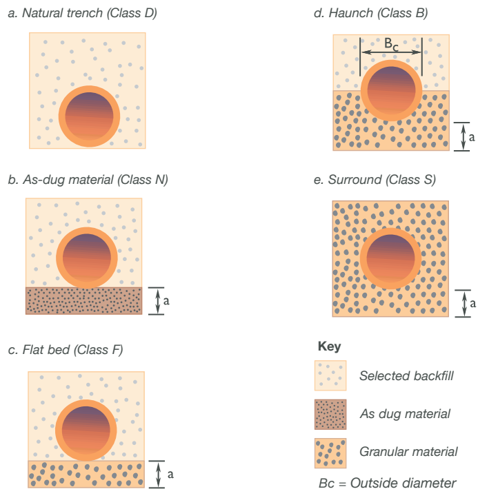
Fig. 5 – Bedding
