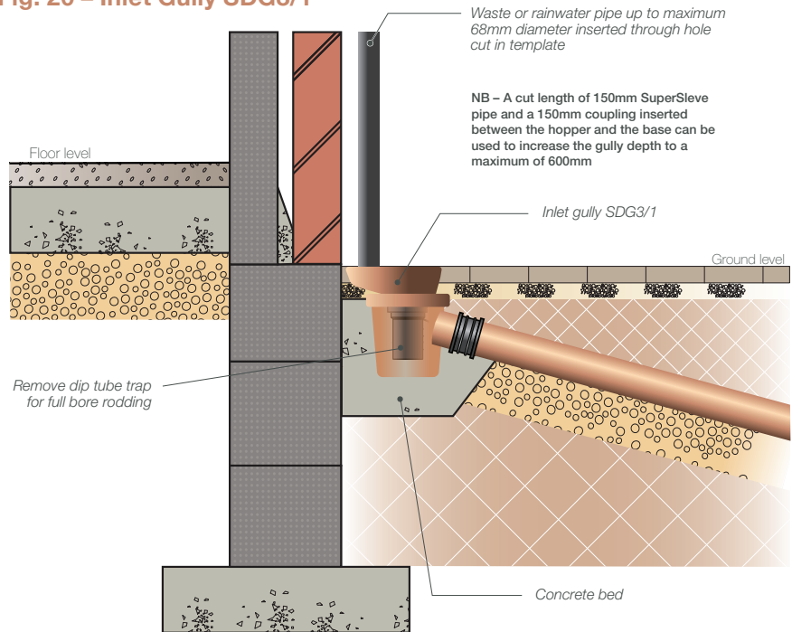
Fig. 20 – Inlet Gully SDG3/1
