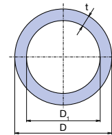
Wavin Ekoplastik PP-R pipe S 5 / PN 10 / SDR 11
