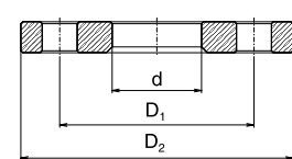
Flange
