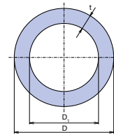
Wavin Ekoplastik PP-R pipe S 3,2 / PN 16 / SDR 7,4
