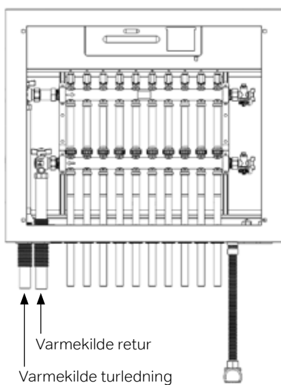
Tilkoblingsskisse venstre
