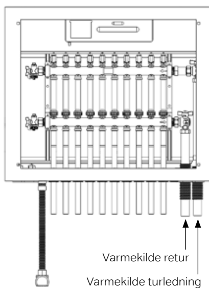
Tilkoblingsskisse høyre
