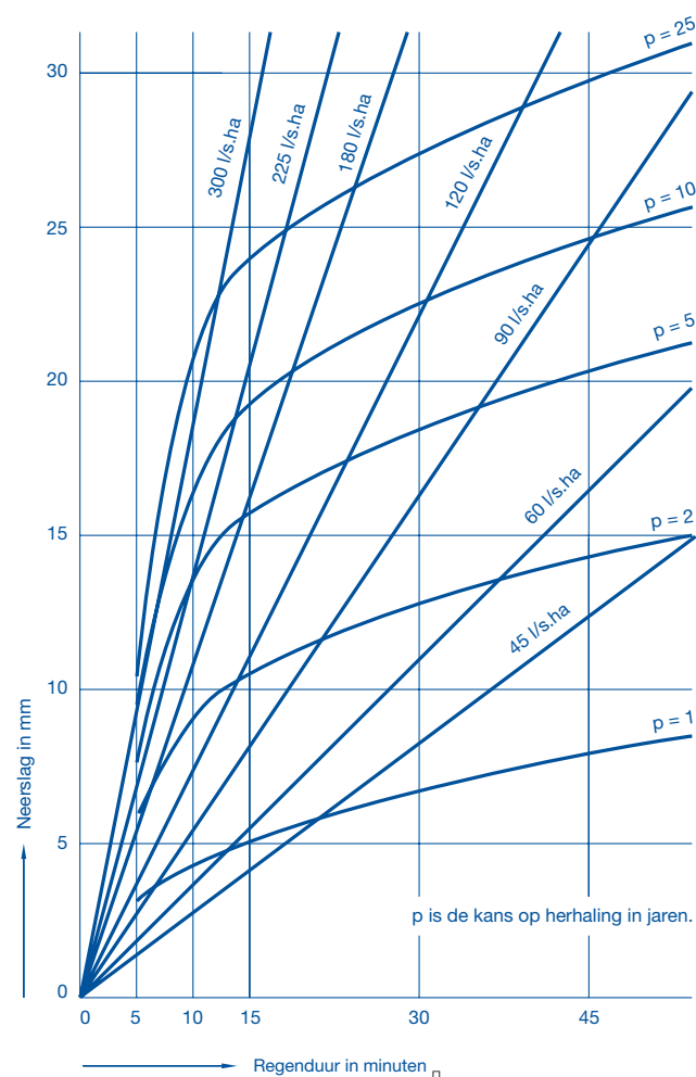
Afb. 6. Regenkurven met kans op herhaling in jaren met diverse ontwerpregenintensiteiten. Bijvoorbeeld: één keer in de vijf jaar komt gedurende 10 minuten een bui voor van 225 l/s.ha
