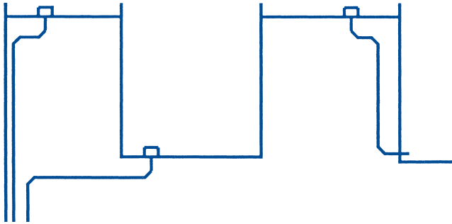
Afb. 10. Afwatering bij ingesloten en op verschillende hoogten gelegen daken. Deze opstelling is ook bruikbaar voor Wavin PE QuickStream-overlatten.
