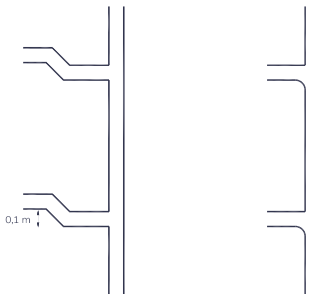
Afb. 4.20. Boven elkaar liggende toiletten moeten worden aangesloten met een sprong van 0,1 m of met stroom T-stukken.
