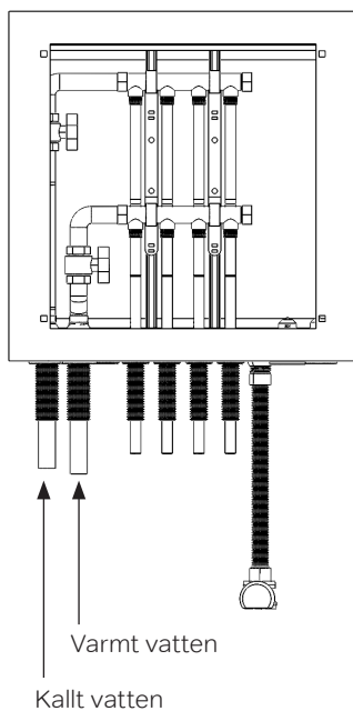
Anslutningsskiss Vänster
