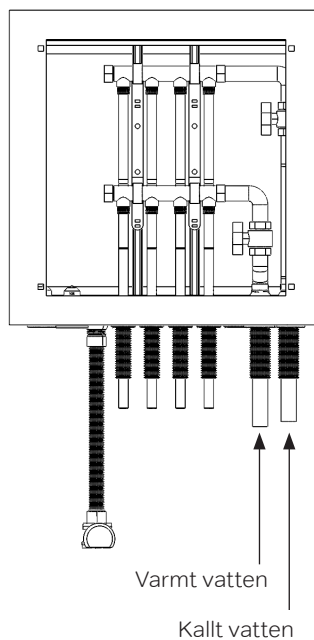
Anslutningsskiss Höger
