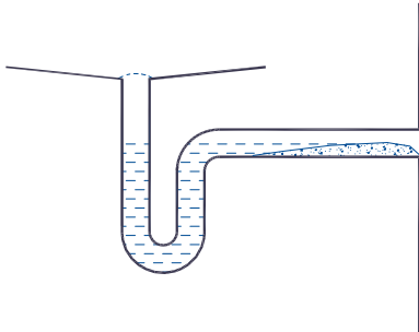
Afb. 4.6. Zonder staand deel in de toestelleiding kan de liggende leiding en de sifon vervuilen
