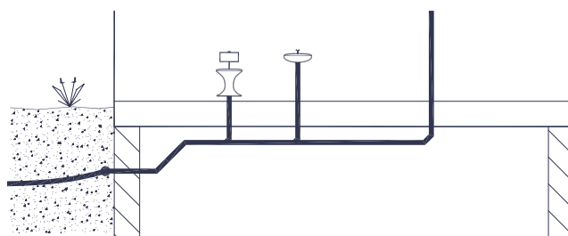
Afb. 4.26. Hang de ondergrondse verzamelleiding zo hoog mogelijk.
