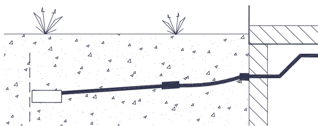
Afb. 4.32. Direct buiten de fundering komt een zettingsconstructie.
