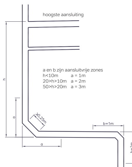
Afb. 4.23. Overgang standleiding/liggende leiding en aansluitvrije zones.
