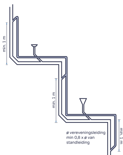
Afb. 4.25. Vereveningsleiding.
