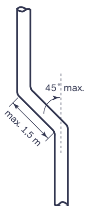
Afb. 4.22. Versleping in de standleiding.
