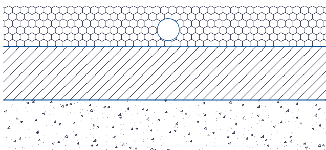
Afb. 4.30. Vloer op zand, leiding opgenomen in isolatie.
