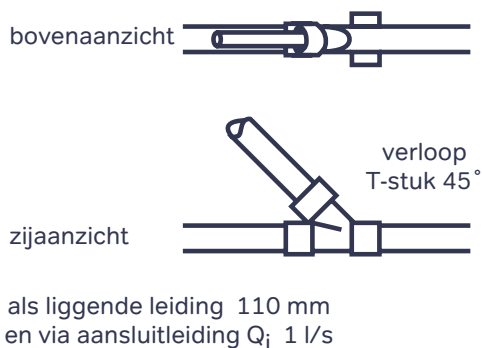
Afb. 4.14. Boven aansluiting.
