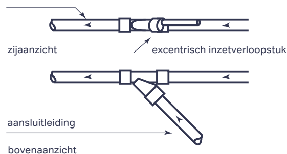
Afb. 4.12. Horizontale aansluiting op verzamelleiding met een excentrisch verloopstuk.
