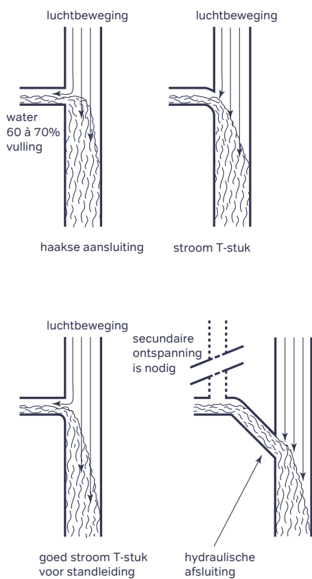
Afb. 4.19. Aansluitingen op de standleiding.
