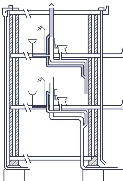
Afb. 4.4. Voorbeelden van een vereveningsleiding.
