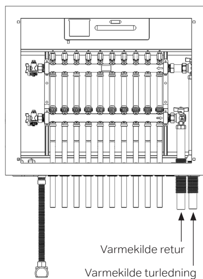
Tilkoblingsskisse højre
