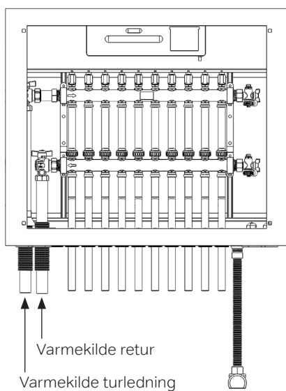
Tilkoblingsskisse venstre
