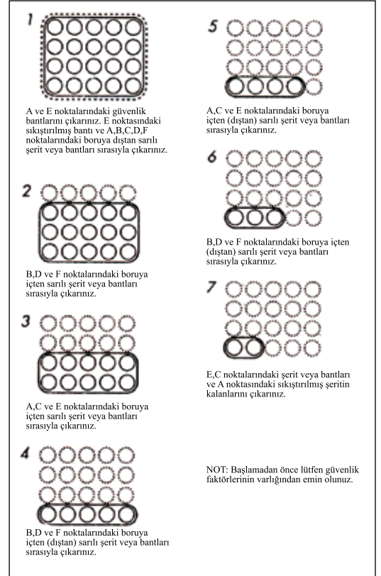
Bantla Sarılı Kangal Boruların Açılması
