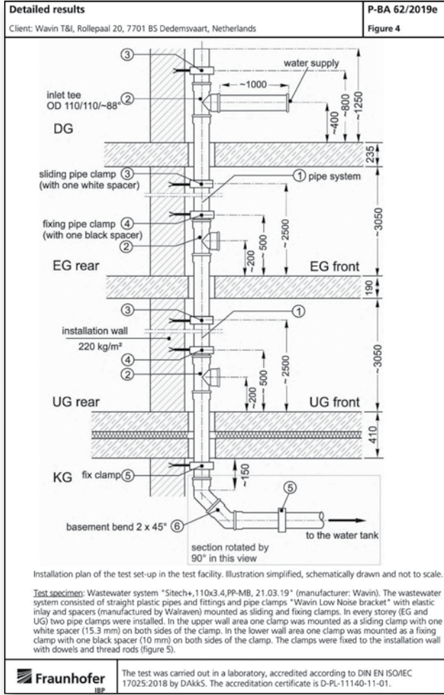
Şekil 3: Laboratuvarda montaj ses düzeyi ölçümü için FRAU-NHOFFER Test düzeneği.
