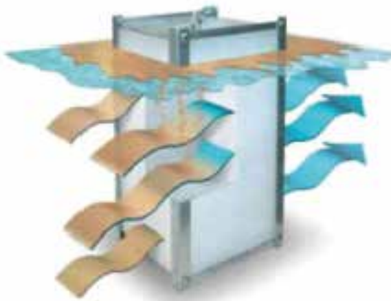
Şekil 4: Koaliser filtre çalışma prensibi
