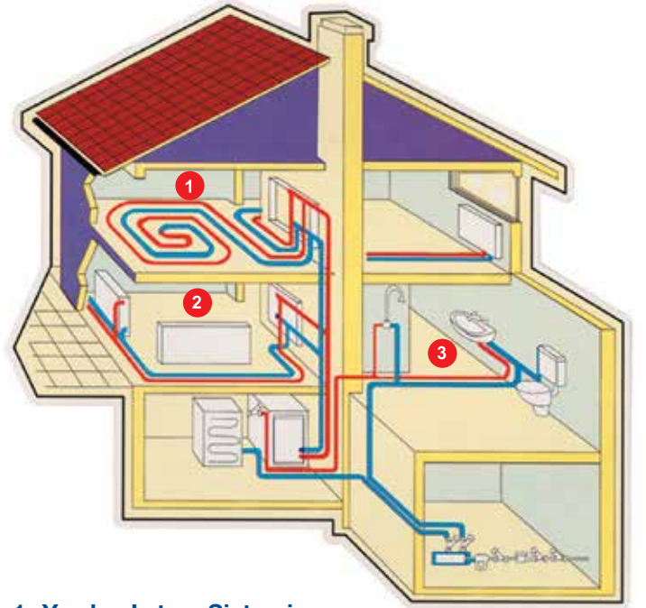
1- Yerden Isıtma Sistemi
