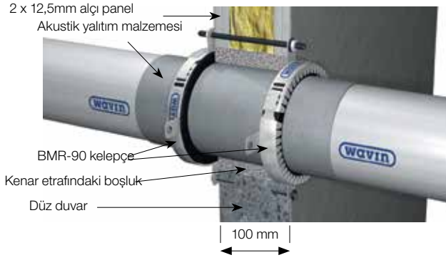
Şekil 24: Manşon/muf olmadan düz montaj.
