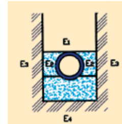
Dik Açılmış Hendek
