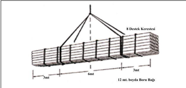
Şekil 2: Çerçeve şeklindeki paketlerin vinç ile taşınması
