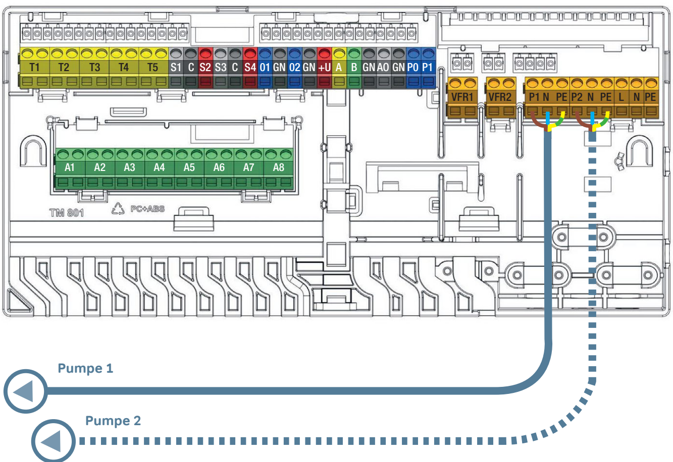
Schaltplan für die Umwälzpumpe(n)
