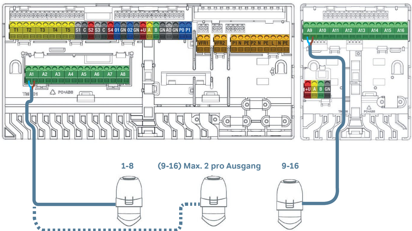
24 V-Stellantriebe anschließen
