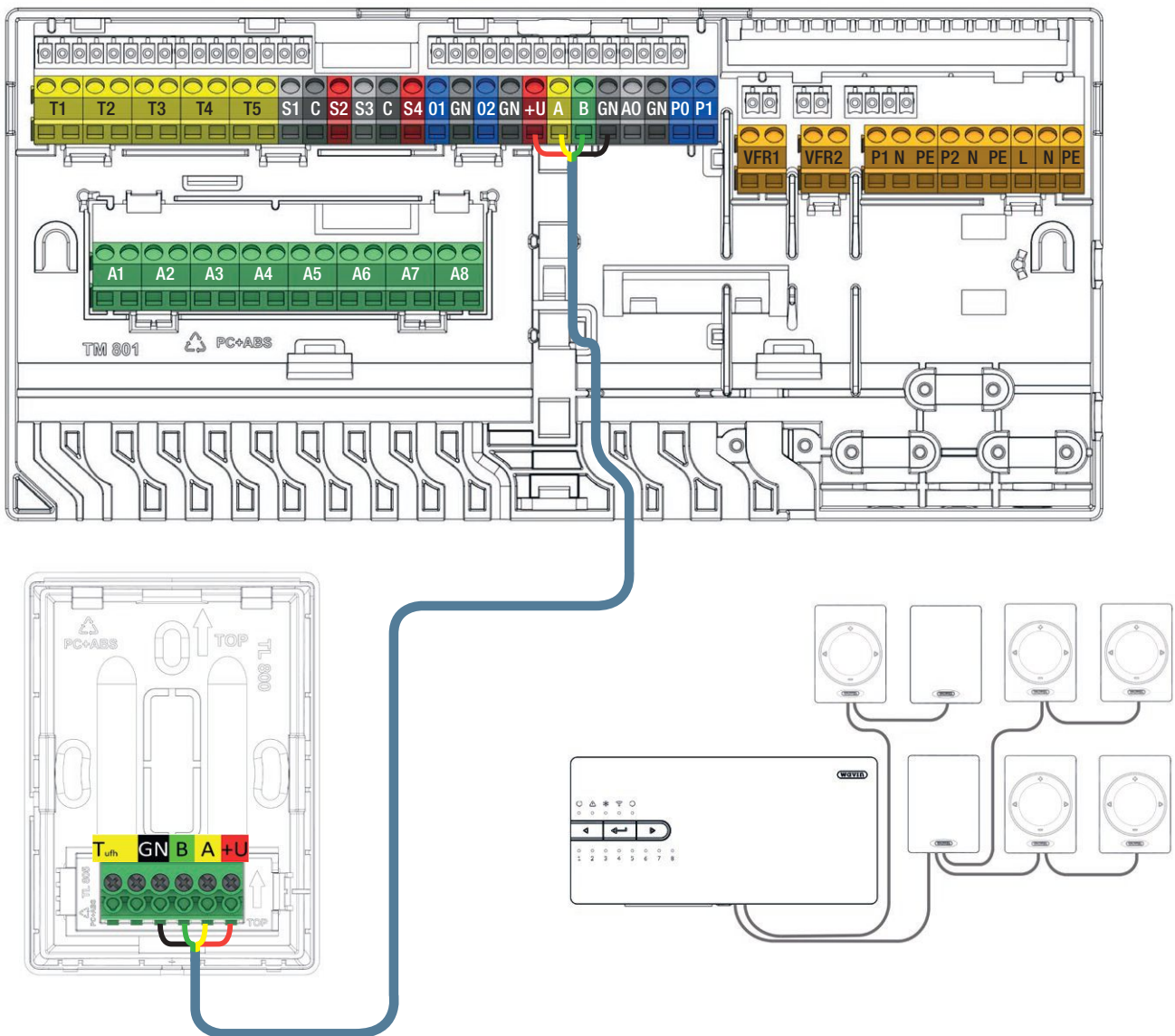
Raumthermostate und Raumtemperatursensoren per BUS-Kabel anschließen
