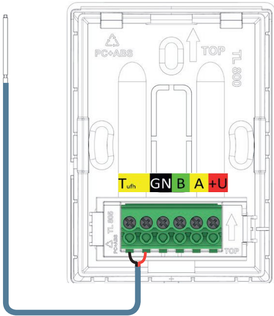
Fußbodensensor mit Kabel anschließen
