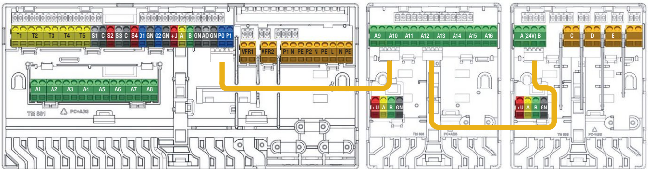
Schaltplan der Verbindungskabel
