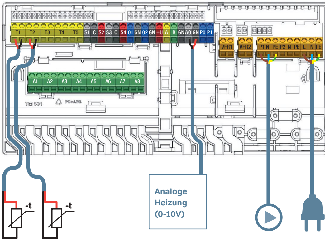
Anschlusschema für Brennwertkessel
