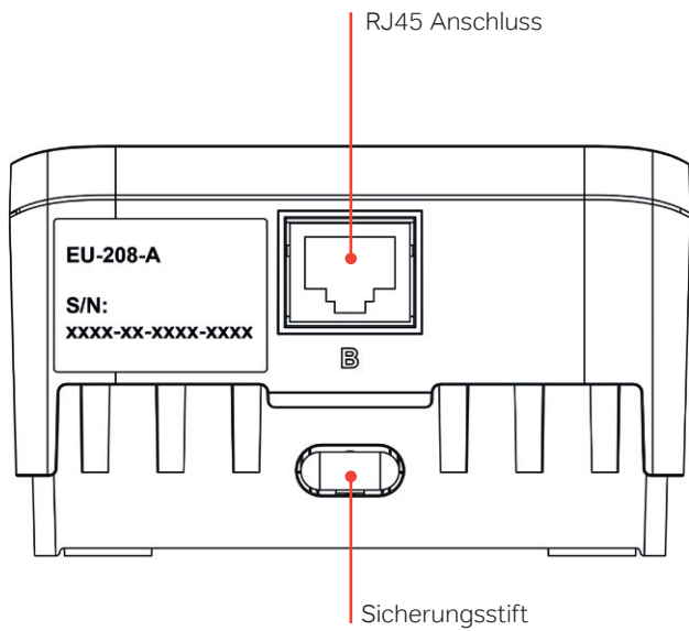
EU Unterseite
