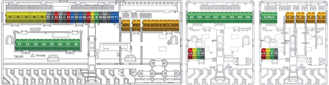
CCU- und EU-Klemmen
