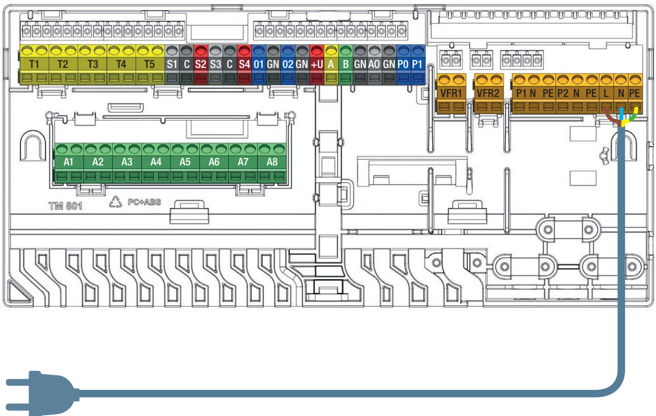
Netzkabel anschließen
