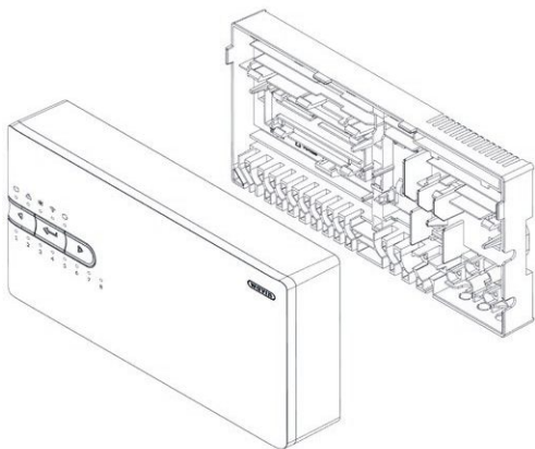
CCU, Explosionszeichnung
