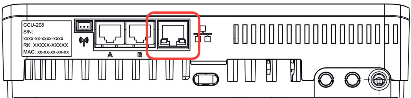
LAN-Verbindung herstellen
