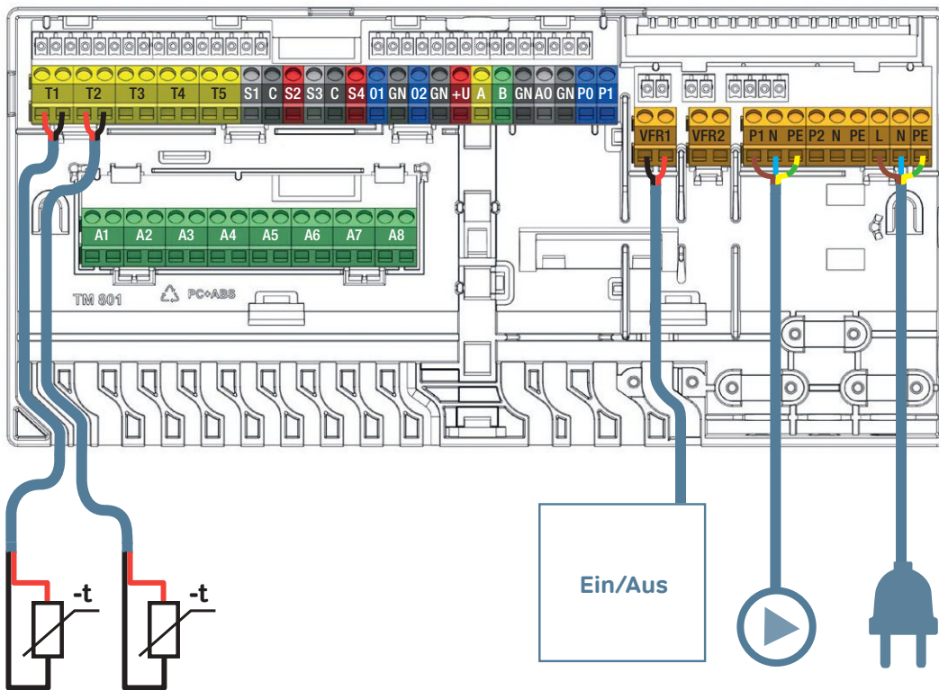
Heizkessel EIN/AUS.
