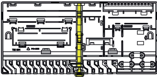
CCU, rückwärtige Platte, mit Sicherungsstift
