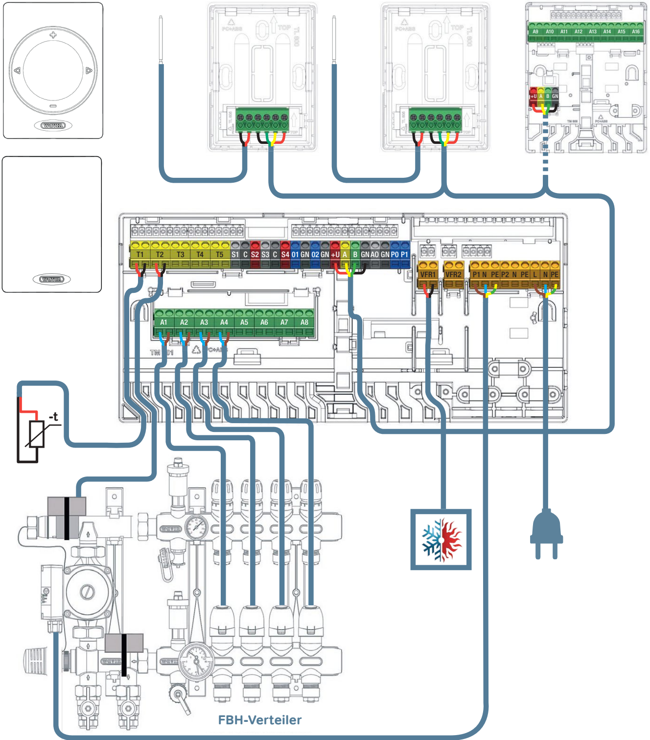
Schaltplan
