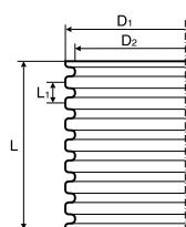
Vsakovací studna DN 1000
