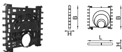
Q-Bic Plus LC deska vstupní 160/400
