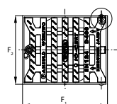
Litínová mříž D400 Ø 315 mm – do teleskopické roury
