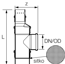
Certaro filtr do šachty
