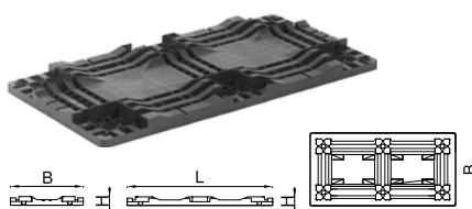
Q-Bic Plus LC dno boxu
