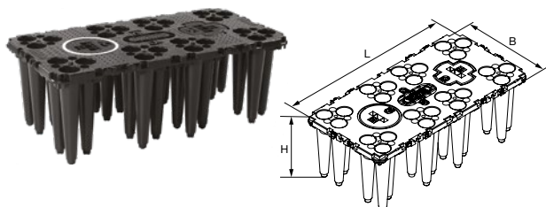
Aquacell NG rPP box akumulární 1,2 x 0,6 x 0,4 m
