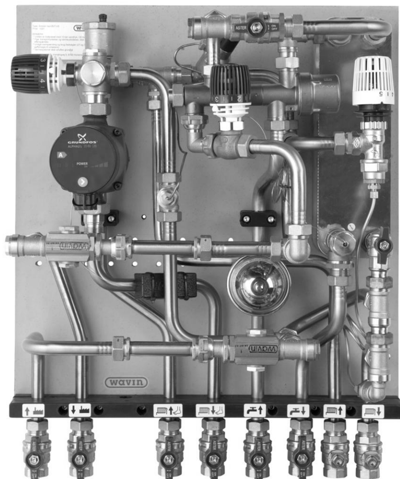
Installationsvejledning for BVT-VS.TD fjernvarmeunit
