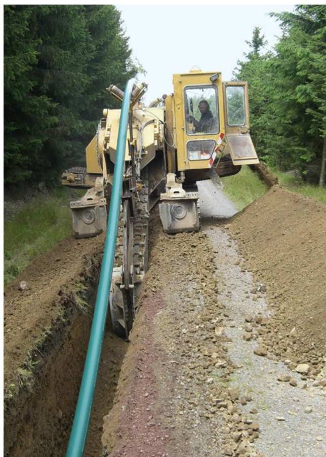
Pokládka kanalizačního potrubí SafeTech RC d140 mm a Wavin TS d140 frézováním v Friedrichsbrunn Harz a Strassberg Harz
