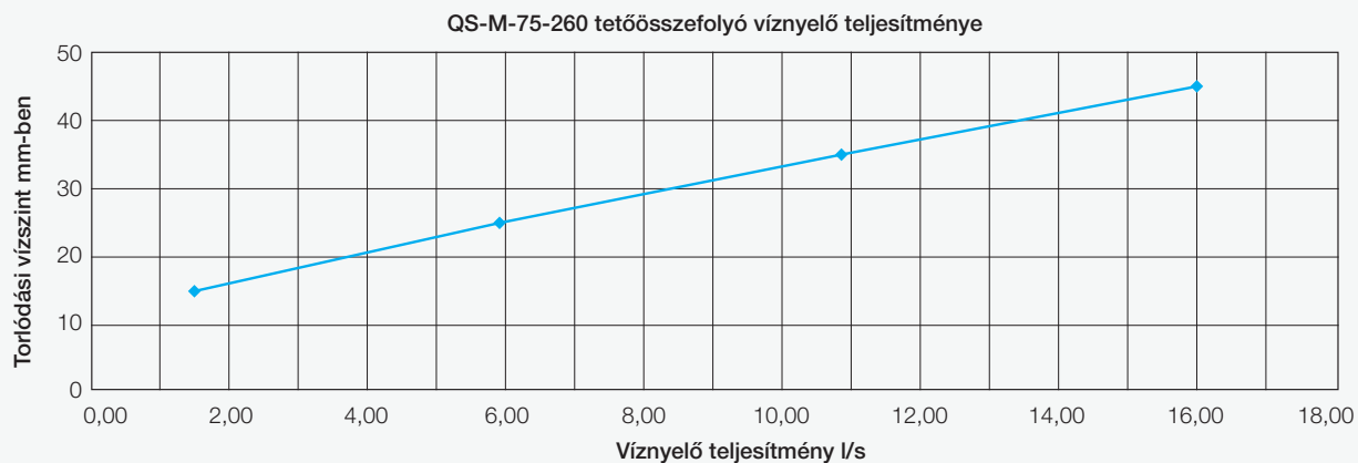
46. ábra: QS-M-75-260 tetőösszefolyó víznyelési teljesítmény grafikonja (DIN EN 1253)
