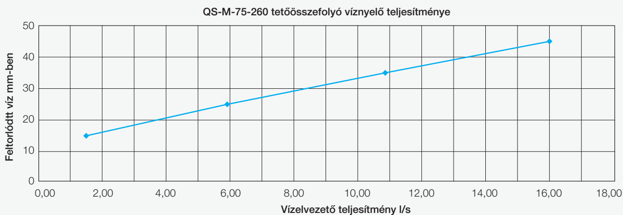
42. ábra: Víznyelési teljesítmény grafikon QS-M-75-260 tetőösszefolyóhoz (DIN EN 1253)
