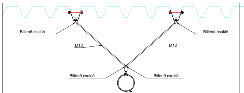
13. ábra: Kikötés acélszerkezethez
