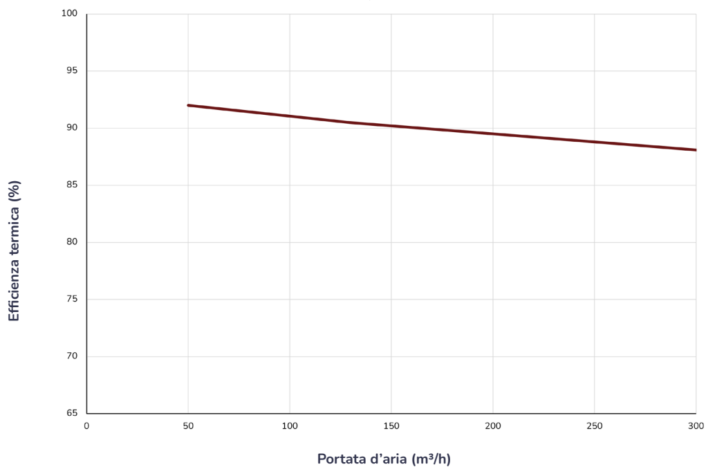
Efficienza termica invernale
