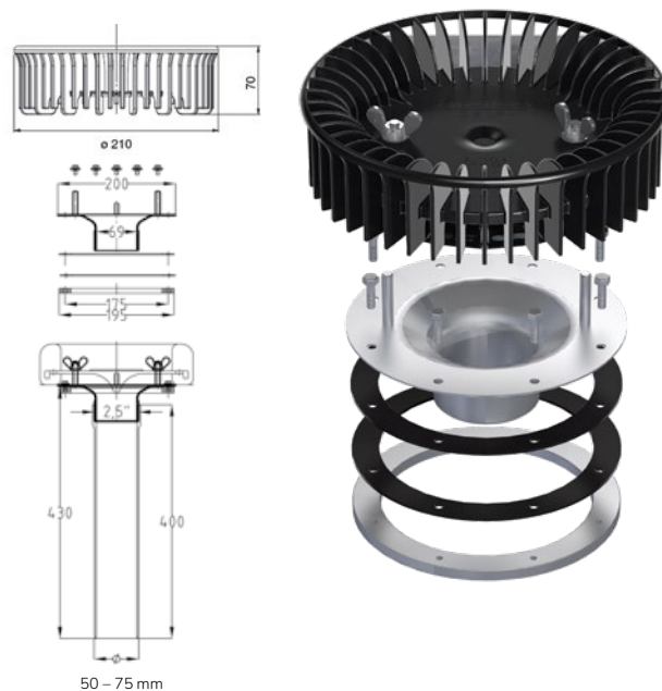
QS-M-200 žlabový typ: Průtok dle DIN EN 1253
