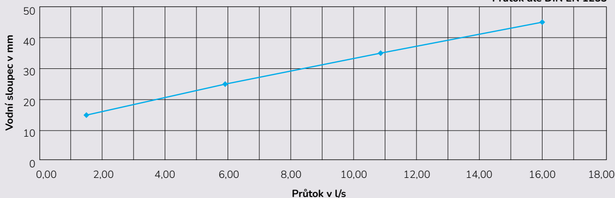
QS-M bitumenový typ + kačirek: Průtok dle DIN EN 1253
