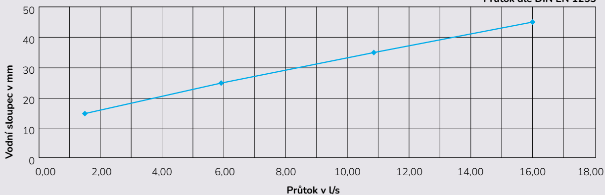
QS-M žlabový typ: Průtok dle DIN EN 1253
