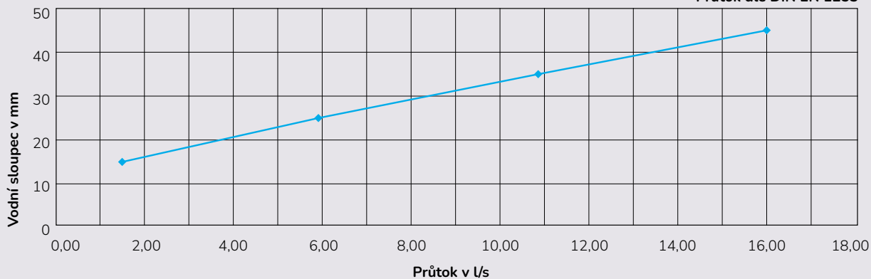
QS-M-200 žlabový typ: Průtok dle DIN EN 1253
