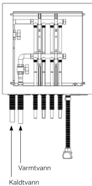
Tilkoblingsskisse venstre
