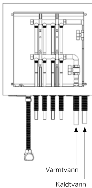
Tilkoblingsskisse høyre
