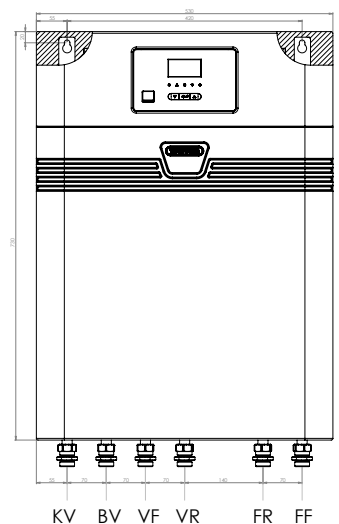
Koblingsdiagram, høyrevendt
