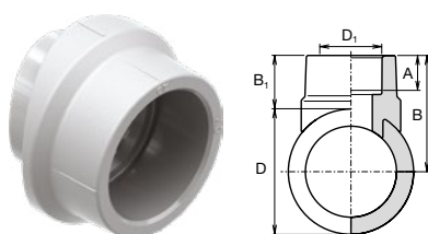
Navařovací sedlo
