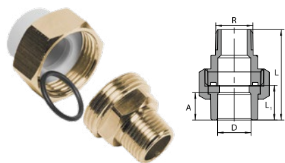
Šroubení hrdlové vnější
