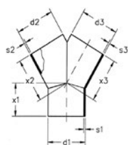
Odbočka Y 30°
