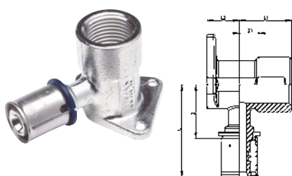
Wavin Tigris M5 – Nástěnné koleno 90° – vnitřní závit prodloužený
