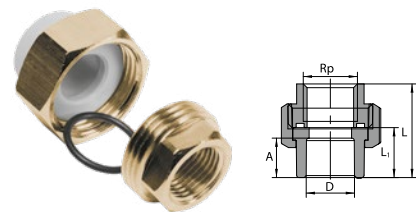
Šroubení hrdlové vnitřní
