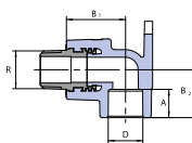
Nástěnné koleno vnější
