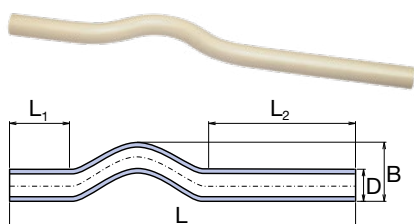
Křížení
