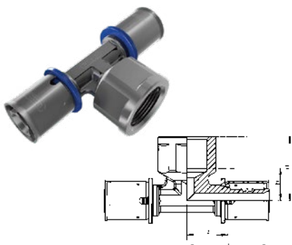
Wavin Tigris M1 – T-kus – vnitřní závit
