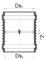
Dvouhrdlá spojka
