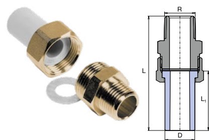
Šroubení vnější
