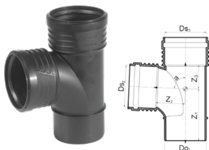
Odbočka se zaoblením
