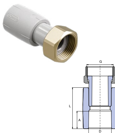
PMD – převlečná matice s dírou pro plombu
