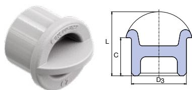
Záslepka vnitřní
