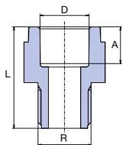
Přechodka s plastovým závitem vnějším
