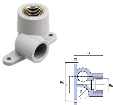
Koncové nástěnné koleno pravé
