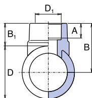
Navářovací sedlo
