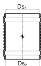
Přesuvka
