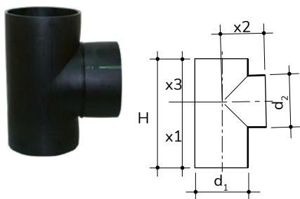
Odbočka 88,5°
