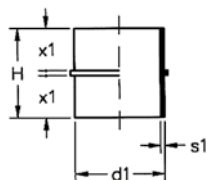
Prstencová objímka
