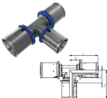
Wavin Tigris M1 – T-kus
