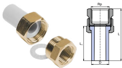
Šroubení vnitřní
