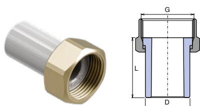
Plastové hrdlo s převlečnou maticí
