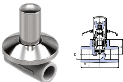
Podomítkový ventil přímý s kovovou krytkou
