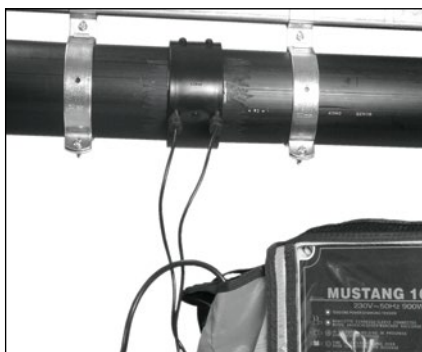
Svařování pomocí elektroodporového nátrubku
