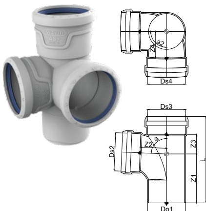
AS+ Odbočka dvojitá rohová 87°
