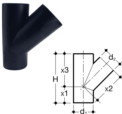
Odbočka 45° – SDR 26
