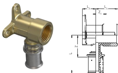
Wavin Tigris M5 – Nástěnné koleno 90° – vnitřní závit
