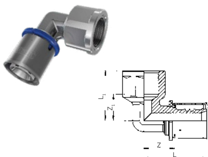
Wavin Tigris M1 – Koleno 90° – vnitřní závit
