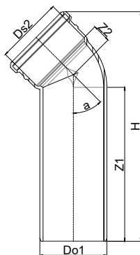
AS+ Koleno prodloužené 45°
