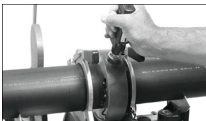
Srovnání konců potrubí integr. hoblíkem
