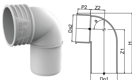
AS+ Připojovací koleno
