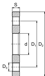
Volná příruba
