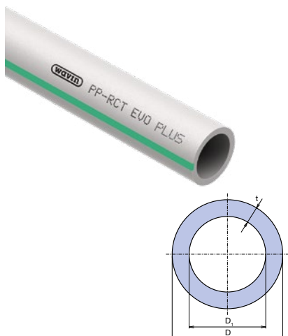
Trubka Wavin PP-RCT EVO PLUS S 3,2 / SDR 7,4 (PN 28 – výpočet)
