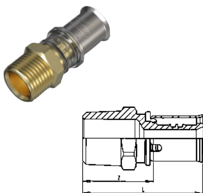
Wavin Tigris M5 – Spojka – vnější závit
