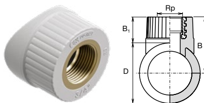
Navařovací sedlo s vnitřním závitem
