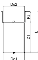
AS+ Připojovací kus
