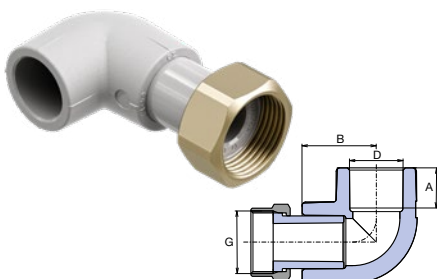
Koleno 90° přechodka plastová s převlečnou maticí
