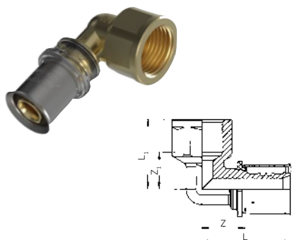
Wavin Tigris M5 – Koleno 90° – vnitřní závit
