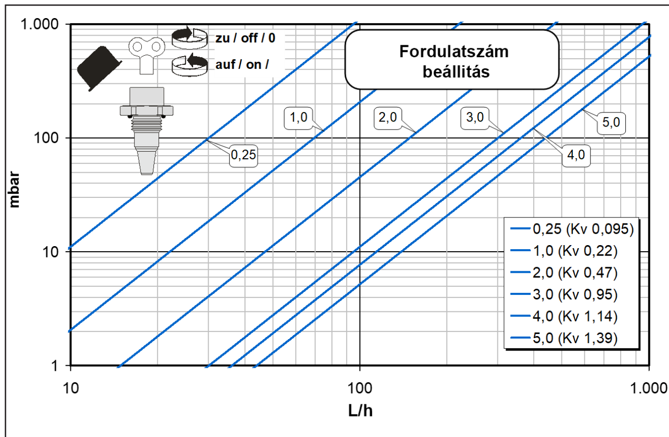
Fig(3): A diagramm az elérhető áramlási sebességet mutatja a szelepfordulatok függvényében
