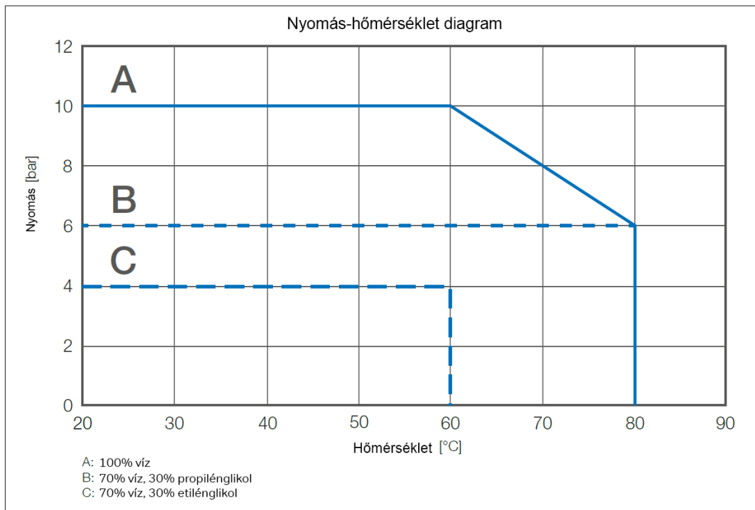
Fig(1): A rendszer előremenő hőmérséklete alapján megengedhető maximális rendszernyomást mutató diagram
