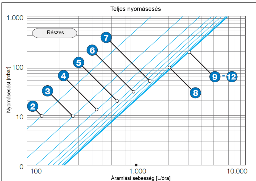
Fig(2): A diagramm a nyomásesést mutatja minden osztó-gyűjtő mérethez az áramlási sebesség függvényében
