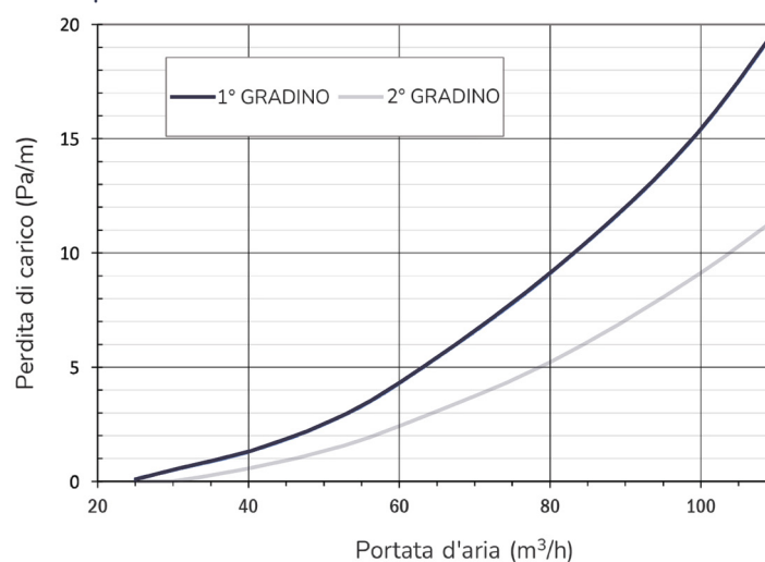
Grafico prestazionale Perdite di carico-Portata d'aria
