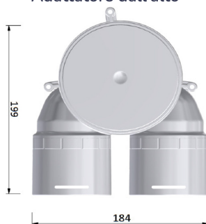
Adattatore dall'alto
