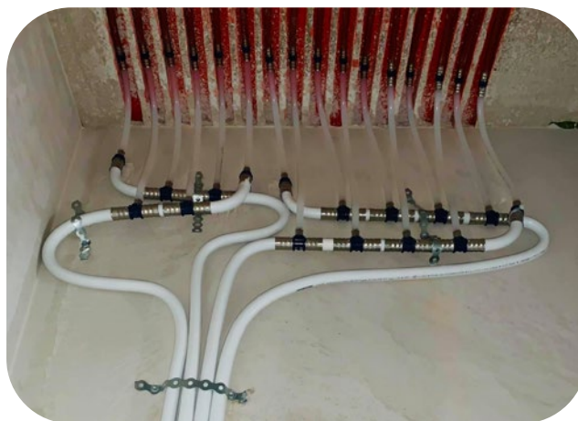
Deska po odstranění bednění s Tichelmannovým připojením vedeným na stěně a připojenými panely Wavin Comfia CW-90
