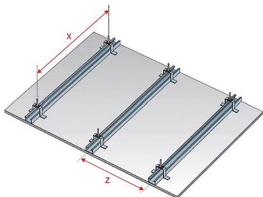
Podhled montovaný přímými kotvami s využitím CD profilů
