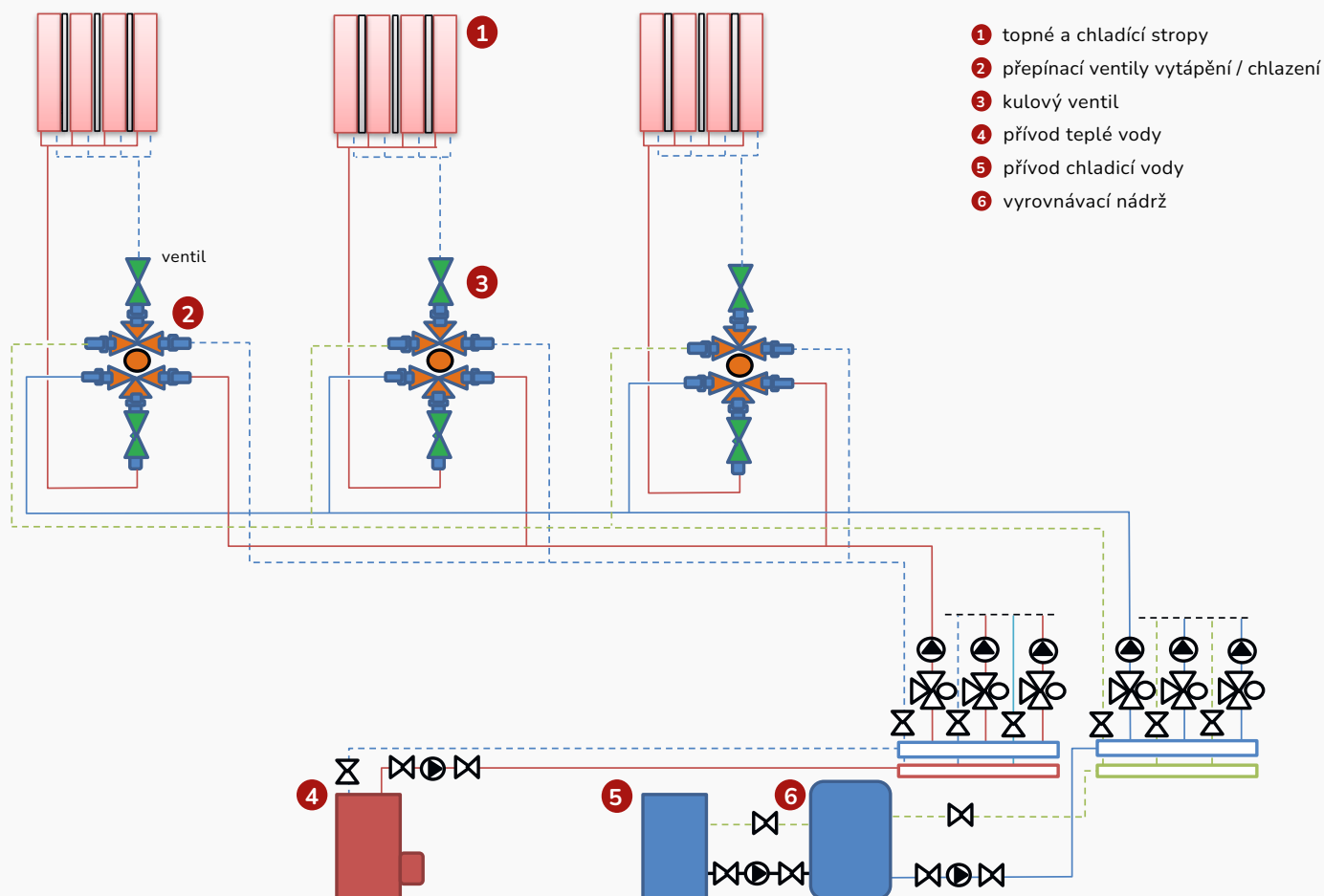
Princip připojení pro chladicí/topný strop ve čtyřtrubkovém režimu
