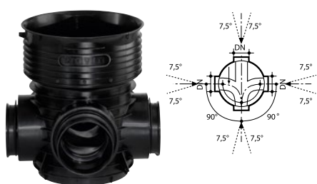
Šachtové dno včetně těsnění – typ X - sběrné 90° (levý i pravý přítok)
