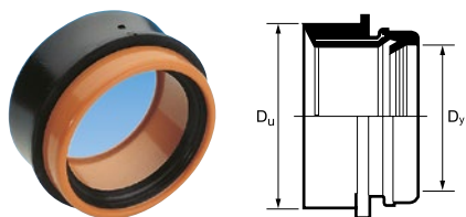
Spojka IN-SITU – včetně pryžové těsnicí manžety
