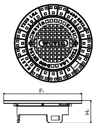
Litinový poklop D400 Ø 315 mm – kulatý do teleskopické roury
