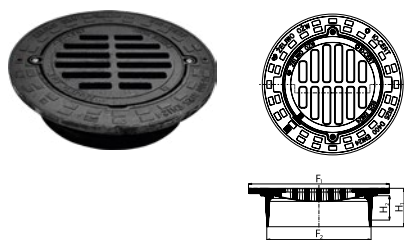
Litinná mříž B125 Ø425 mm – do teleskopické roury
