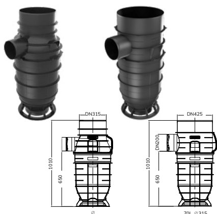
Uliční vpust Tegra se sifonem a filtrem
