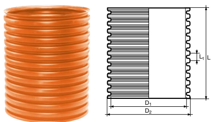
Šachtová vlncová roura SN4
