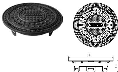
Litviný poklop B125 Ø 425 mm – kulatý do teleskopické roury
