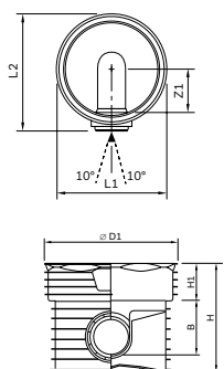
Šachtové dno včetně těsnění – koncové
