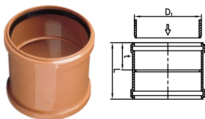
KG PVC-U - Spojka dvouhrdlá
