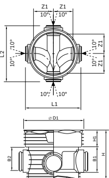
Šachtové dno včetně těsnění – typ X - sběrné 90° (levý i pravý přítok)
