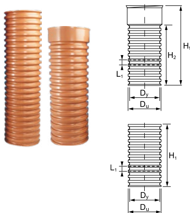
Šachtová korugovaná roura pro šachtu Basic 315 – s hrdlem, bez hrdla
