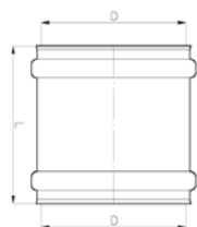
Solidwall PVC SN12 - Přesuvka
