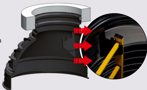
Horní podpora žebříku – konzola pro zachycení žebříku v konusu
