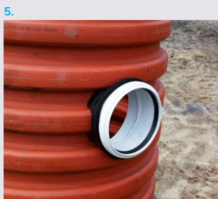
Vnitřek instalovaného těsnění se maže kluzným prostředkem, což umožňuje vsunutí potrubí.
