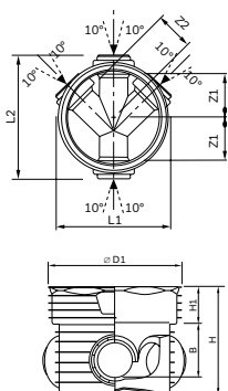
Šachtové dno včetně těsnění - typ Y -sběrné 45°
