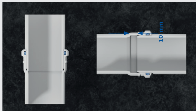
Bild. 28: Säkerställ 10 mm i expansionsutrymme.
