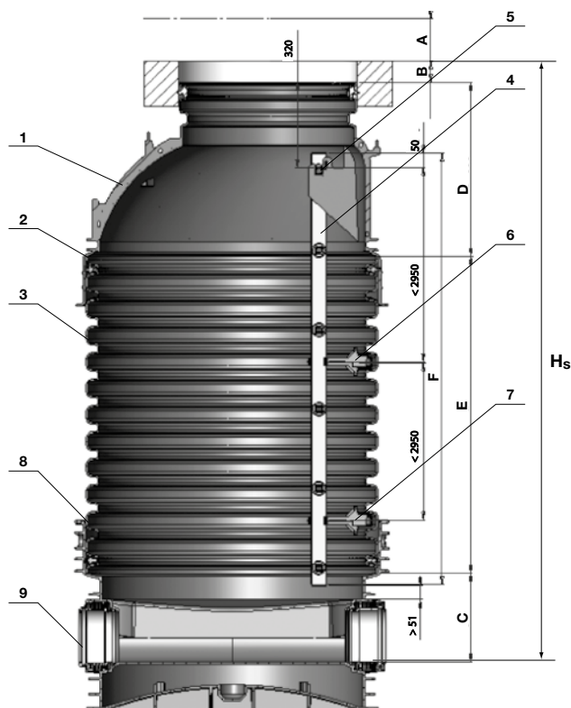
Schemat montażowy studzienki Tegra 1000.
