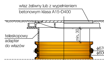
Wąż A15, B125 lub D400 na teleskopowym adapterze do wążów
