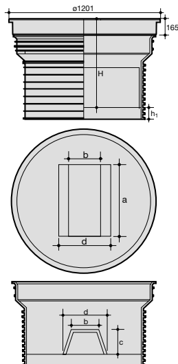
Komora pomiarowa Tegra 1000 z cokołem
