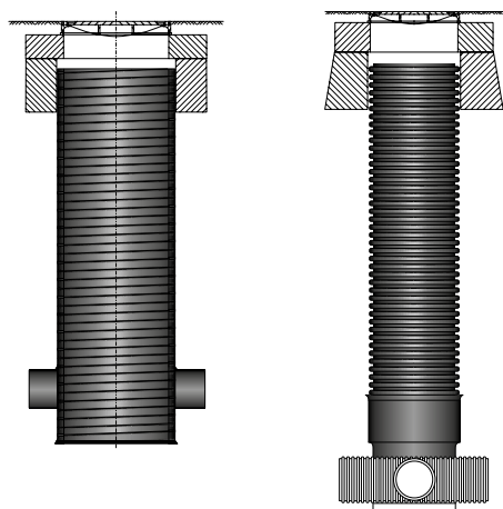
Rys. 1: Przykładowe rozwiązania studzienek z kietą przepływową wykonane z rur strukturalnych:
