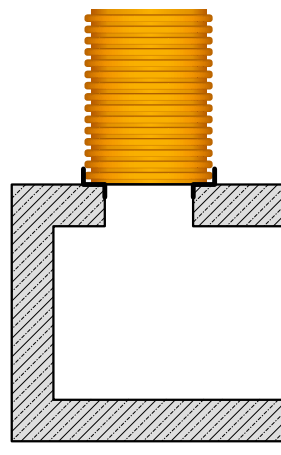
Rys. 4: Przykładowe rozwiązanie studzienek – nadstawka: szyb włazowy lub inspekcyjny do zbiornika.
