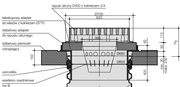
Wpust uliczny lub z żeliwa szarego na teleskopowym adapterze z kołnierzem DN 770
