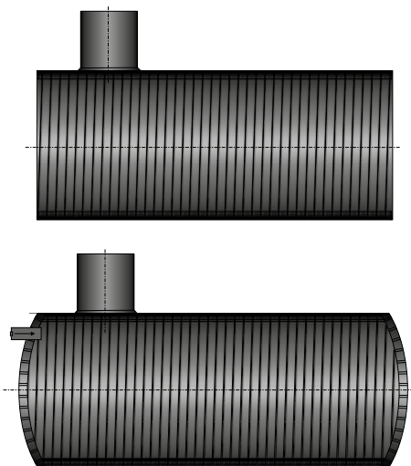
Rys. 3: Przykładowe rozwiązanie studzienek – zbiorników poziomych wykonanych z rur strukturalnych.
