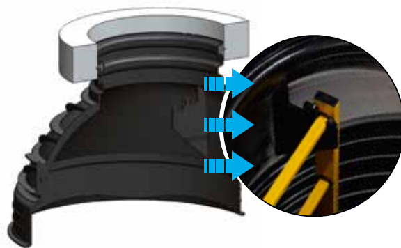
Rys. 3: Szczegół – górne wsparcie drabinki – uchwyt drabinki usytuowany w stożku.
