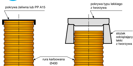
Pokrywa A15 na rurze karbowanej
