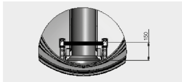
Usytuowanie szczelki drabinki w świetle otworu włazowego stożka – widok z góry.
