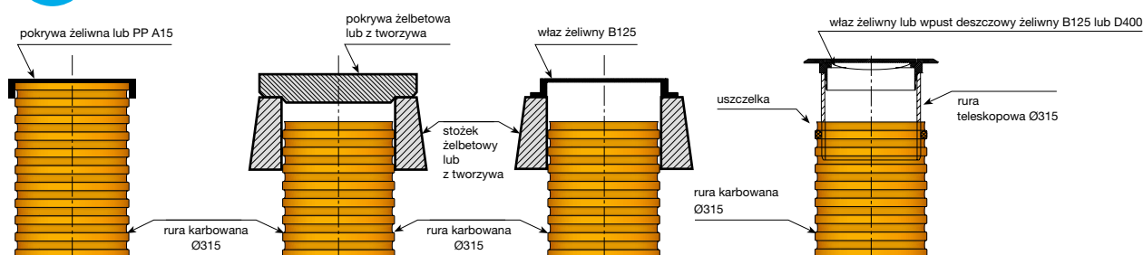
Pokrywa A15 na rurze karbowanej
